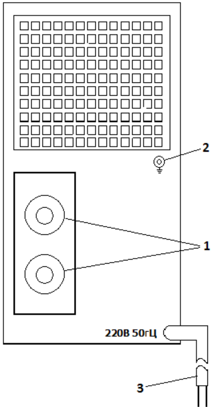
Рис.1. Задняя панель комплекта СИЛУС-Т 1600А
