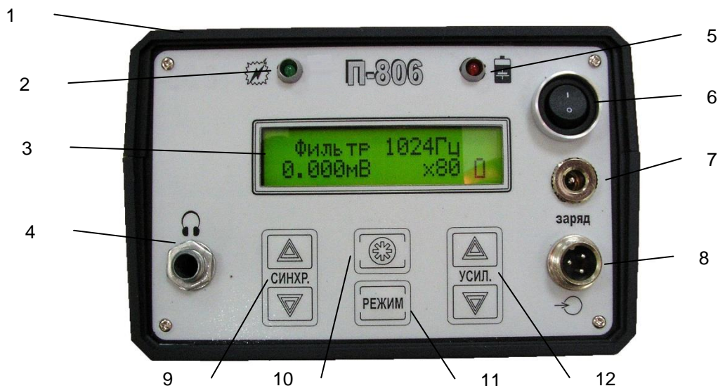
Рисунок 1. Приемник П-806. Вид передней панели.
