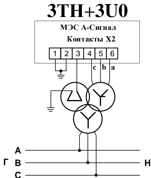
Рисунок 2.5 Вариант схемы подключения ЗТН+ТННП
