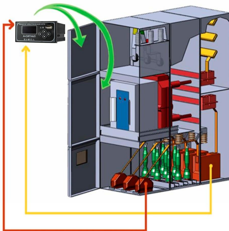
Рисунок 3. Установка Прибора в ячейке КРУ
