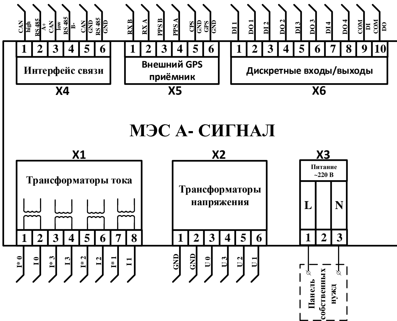
Рисунок 2.1 Схема подключения Прибора
