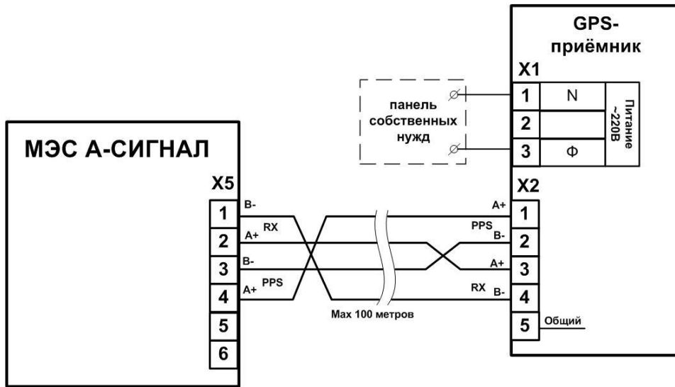
Рисунок 2.8 Схема подключения GPS-приёмника к Прибору
