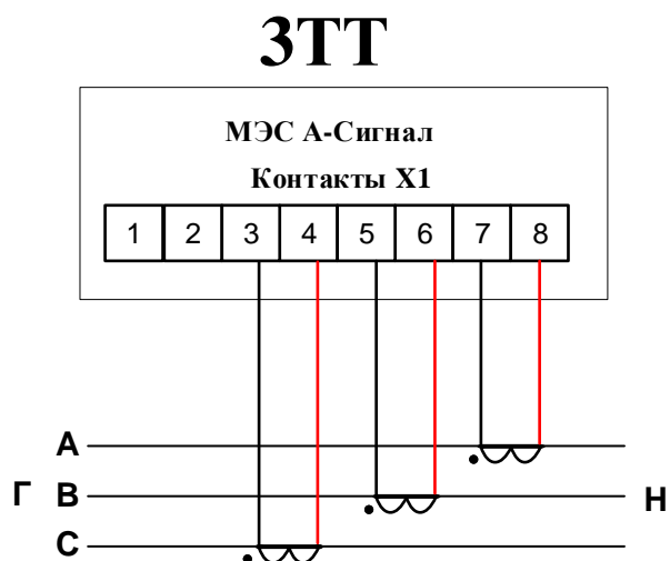
Рисунок 2.4 Вариант схемы подключения ЗТТ
