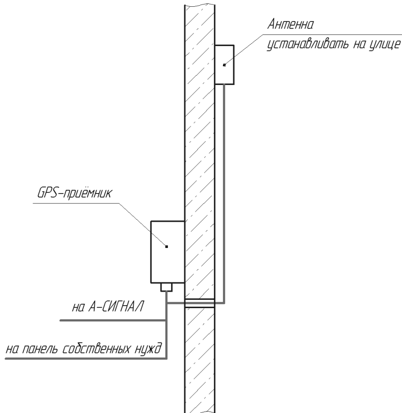
Рисунок 2.8 Схема подключения GPS-приёмника к Прибору
