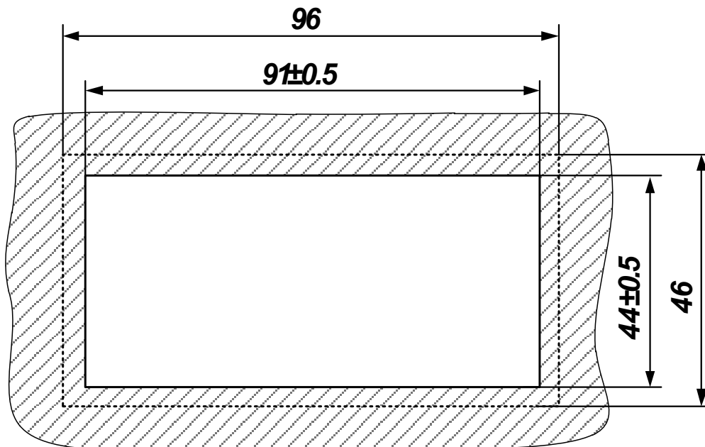
Рисунок 2.15 Размеры вырубного отверстия в щите для установки А-СИГНАЛА
