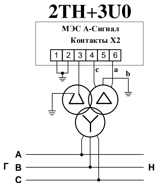
Рисунок 2.7 Вариант схемы подключения Прибора
