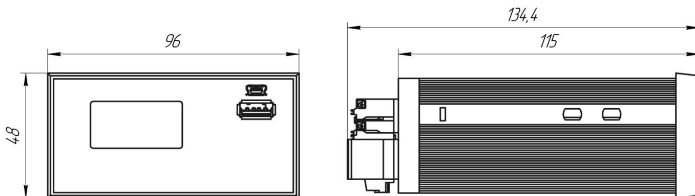
Рисунок 1.1 Габаритные размеры Прибора
