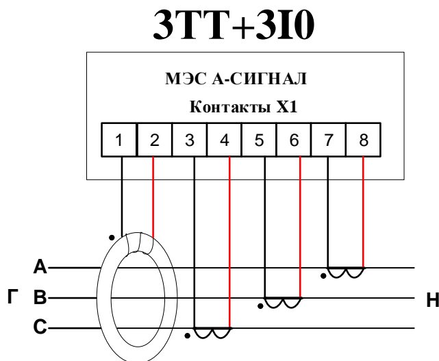
Рисунок 2.2 Вариант схемы подключения 3ТТ+ТТНП.
