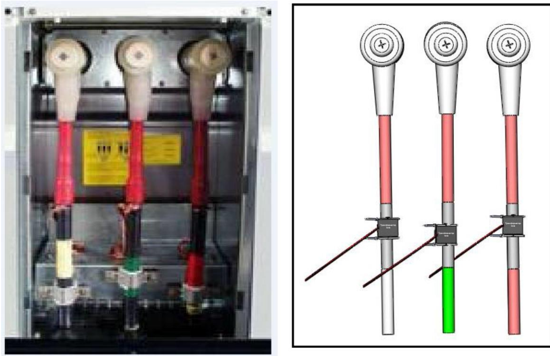
Рисунок 2.12 – Трансформатор тока устанавливается на каждый кабель
