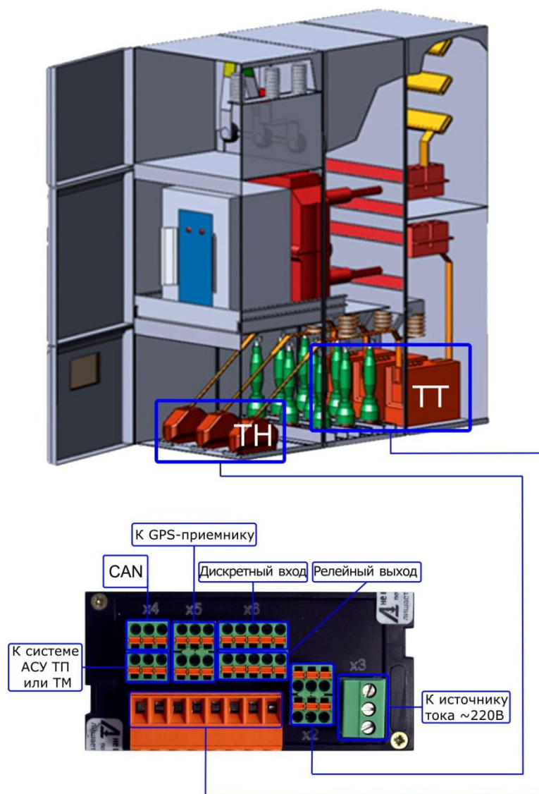
Рисунок 4 – Подключение Прибора
