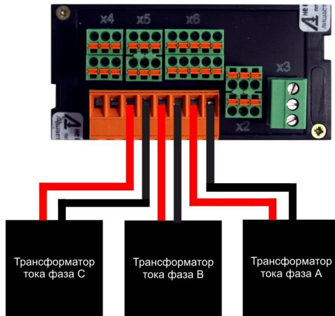
Рисунок 2.14 – Схема подключения ТТ к Прибору
