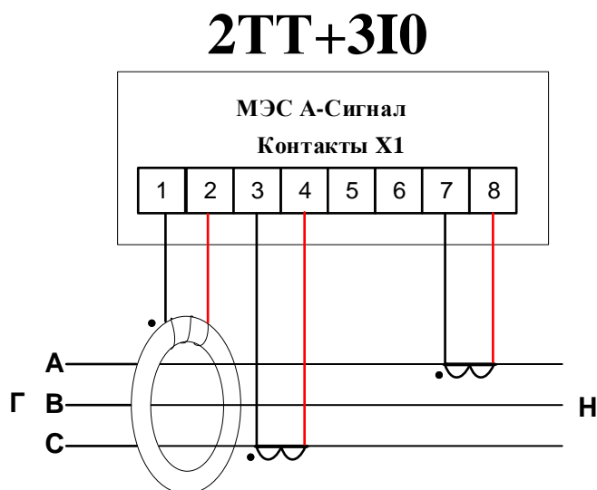
Рисунок 2.3 Вариант схемы подключения 2ТТ+ТТНП
