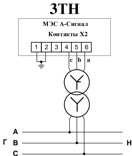
Рисунок 2.6 Вариант схемы подключения 3 ТН
