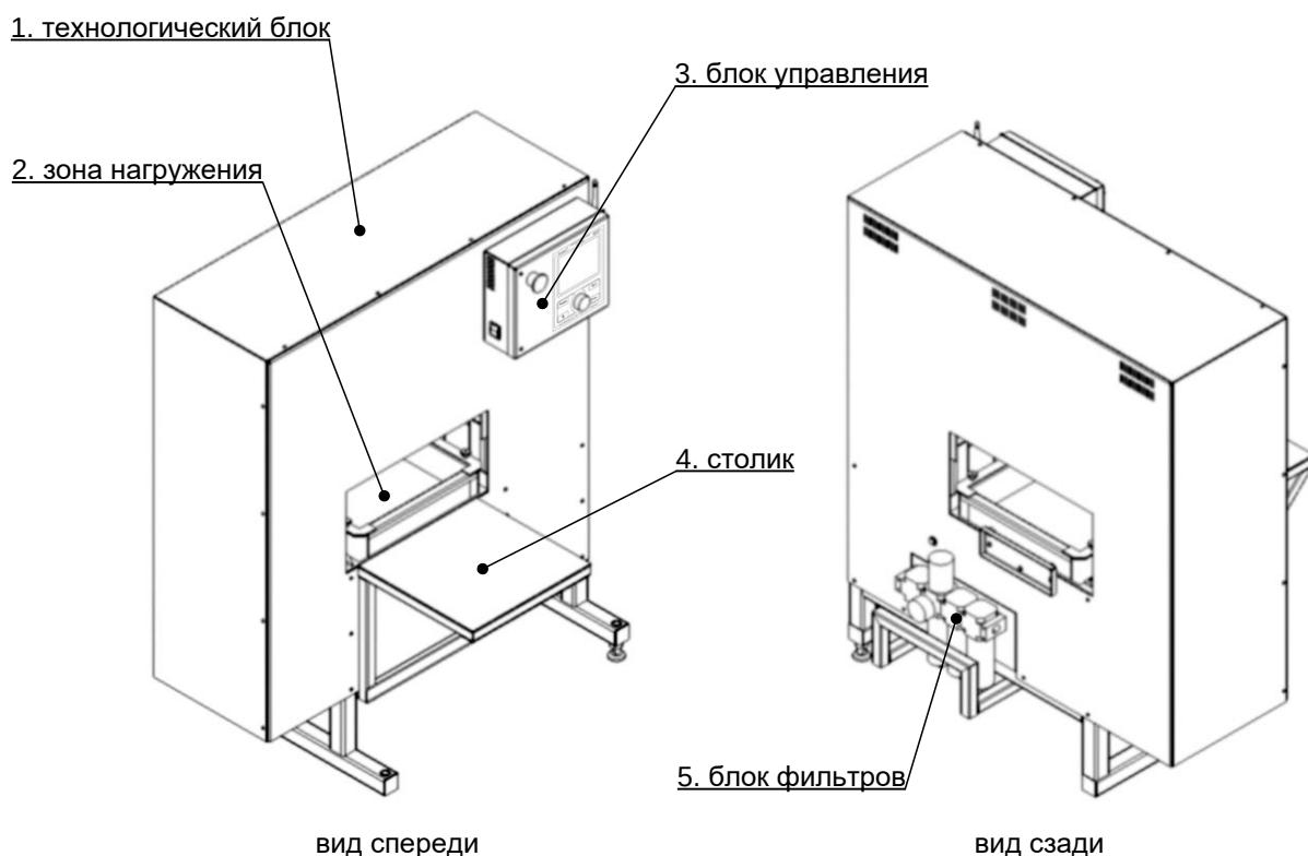
Рисунок 1 – Общий вид аппарата
