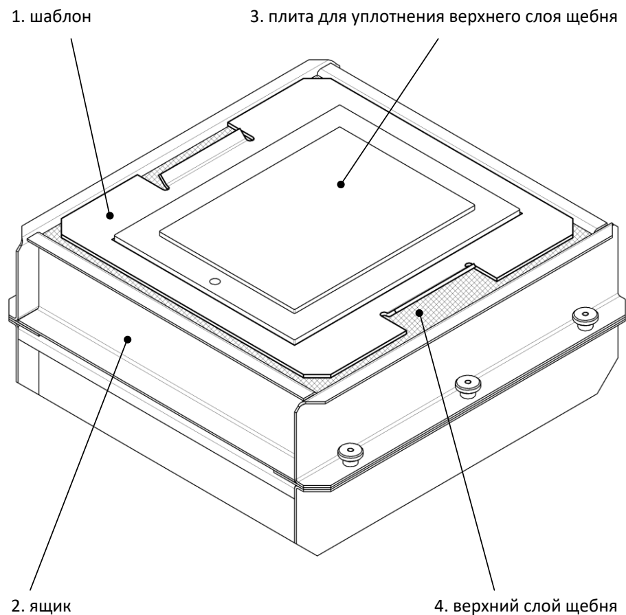
Рисунок 9 – Уплотнение верхнего слоя щебня
