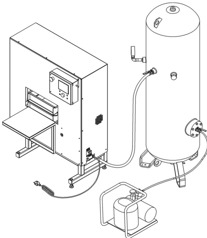
Рисунок 5 – Монтажная схема
