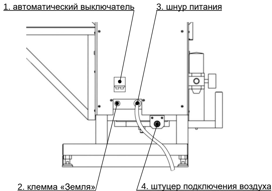
Рисунок 3 – Узел подвода питания
