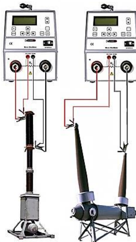
Рисунок 3 – Подключение к выключателю
