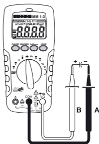
BENNING MM 1-2/ 1-3 Bild 9: Kapazitätsmessung Fig. 9: Capacity testing Fig. 9: Mesure de capacité Fig. 9: Medición de capacidad obr. 9: Měření kapacity figur 9: Kapacitansmåling σχήμα 9: Μέτρηση χωρητικότητας 9. ábra: Kapacitás mérés ill. 9: Misura di capacità Fig. 9: Capaciteitsmeting Rys.9: Pomiar pojemności Imaginea 9: Măsurarea capacității рис. 9: Измерение емкости Resim 9: Kapasite Ölçümü
