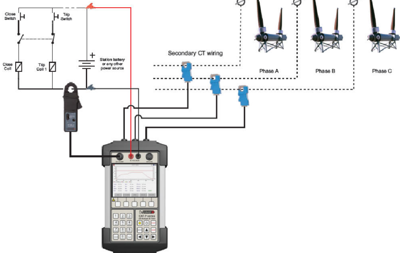
Подключение к тестируемому объекту. ( Фаза А, Фаза В, Фаза С) для онлайн теста
