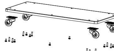
Указания по монтажу роликов
