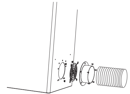
Указания по монтажу трубки-глушителя
