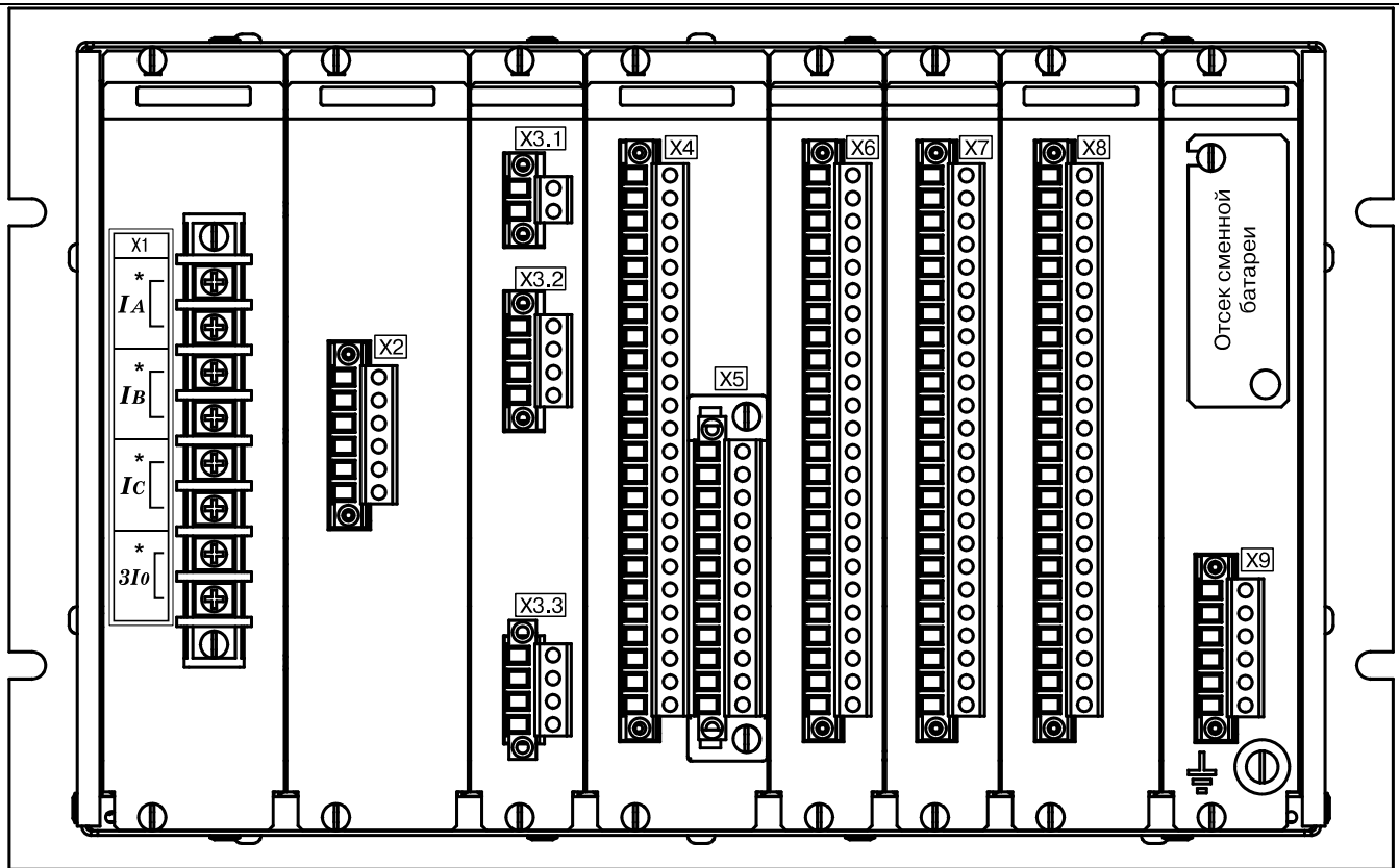
Рисунок Г.4 – Расположение элементов на задней панели устройства «Сириус-2-М»
