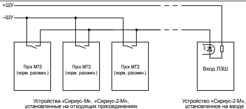
Рисунок Д.5 – Схема соединения нескольких устройств между собой при организации логической защиты шин (параллельная схема)
