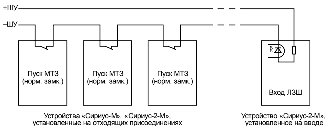
Рисунок Д.6 – Схема соединения нескольких устройств между собой при организации логической защиты шин (последовательная схема)
