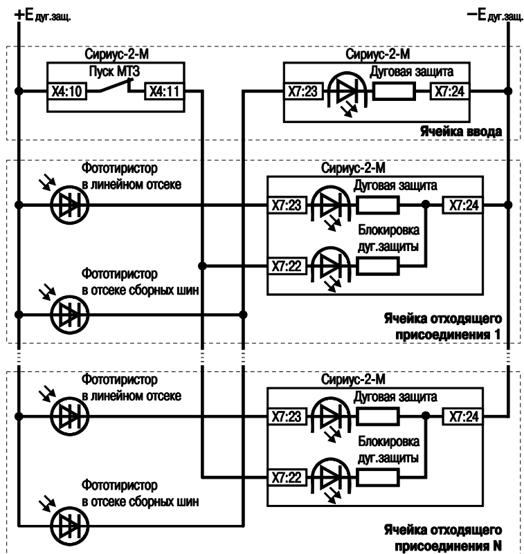
Рисунок Д.7 – Упрощенная схема организации дуговой защиты с использованием контроля по току от защиты вводного выключателя
