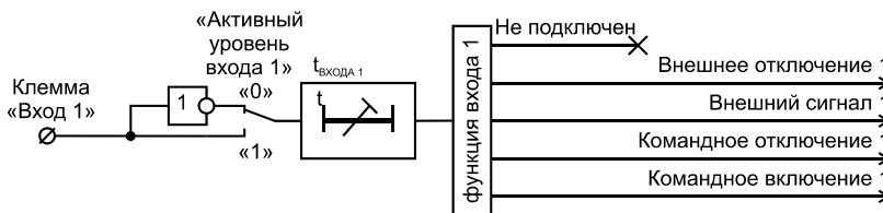
Рисунок И.2 – Фрагмент функциональной логической схемы программируемого входа
