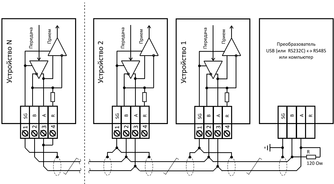
Рисунок Д.4 – Схема подключения устройств с интерфейсом RS485 в локальную сеть. Внешний резистор R устанавливается при отсутствии встроенного резистора.
