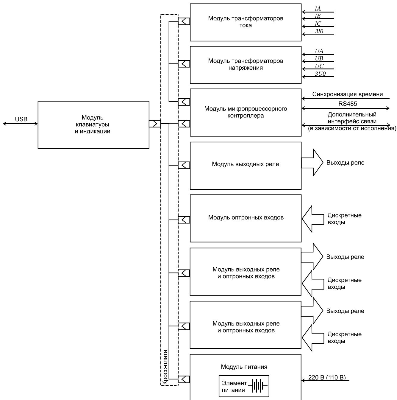
Рисунок 2 – Структурная схема устройства
