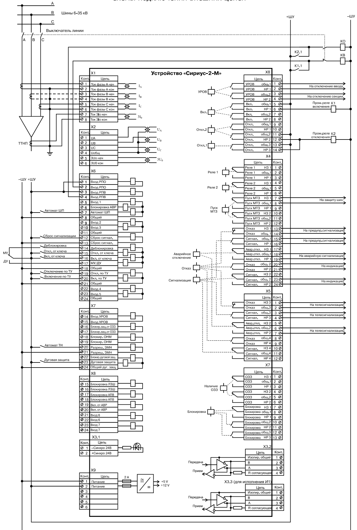
Рисунок Д.1 – Схема подключения внешних цепей к устройству «Сириус-2-М»
