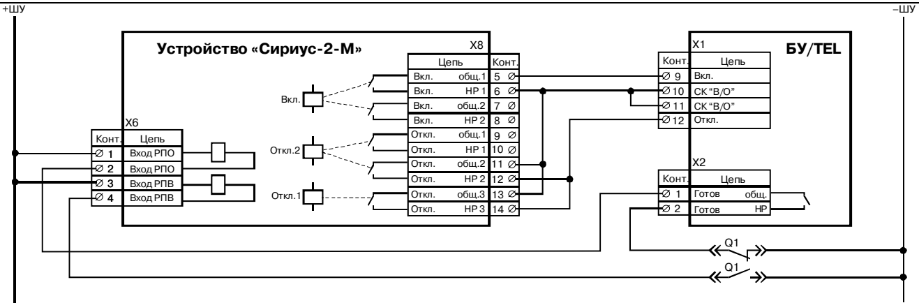
Рисунок Д.2 – Схема подключения устройства «Сириус-2-М» к выключателю ВВ/ТЕЛ с блоком управления БУ/ТЕЛ-12
