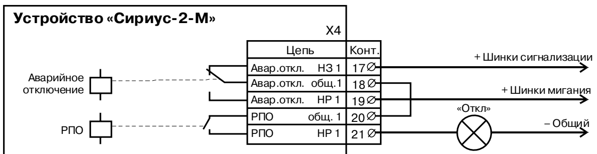
Рисунок Д.3 – Вариант реализации схемы с миганием сигнальной лампочки аварийного отключения устройства с использованием общеподстанционной схемы сигнализации
