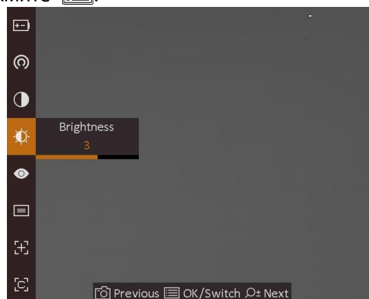
Рис. 2-7. Интерфейс меню
