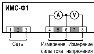
Рисунок 5.1 – Назначение клеммника
