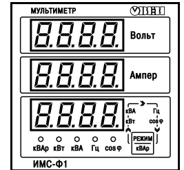
Рисунок 6.2 – Лицевая панель
