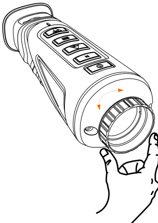
Рисунок 3-3. Регулировка объектива
