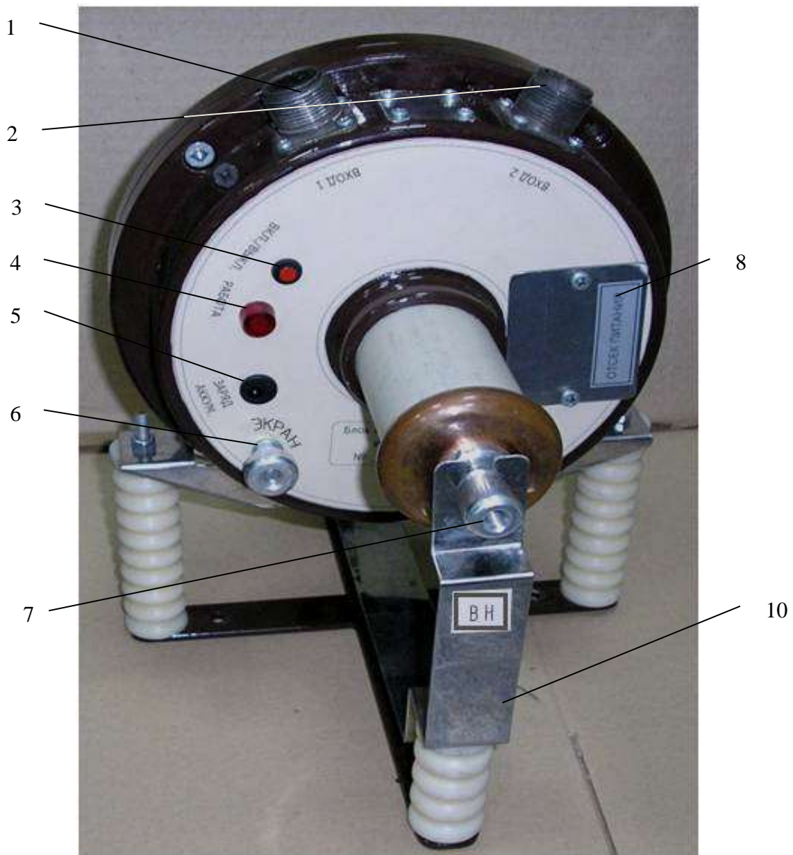
Рисунок 2 Блок высоковольтный ИПИ-10-БВ. Внешний вид.
