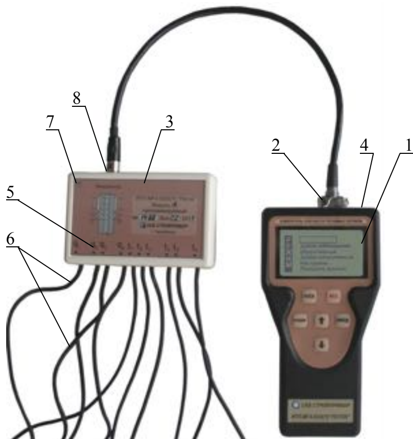
Рисунок 1.1 – Общий вид измерителя ИТП-МГ4.03/10(І) «ПОТОК»
