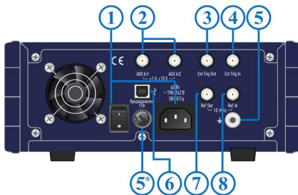
Рисунок 4.4 Задняя панель
