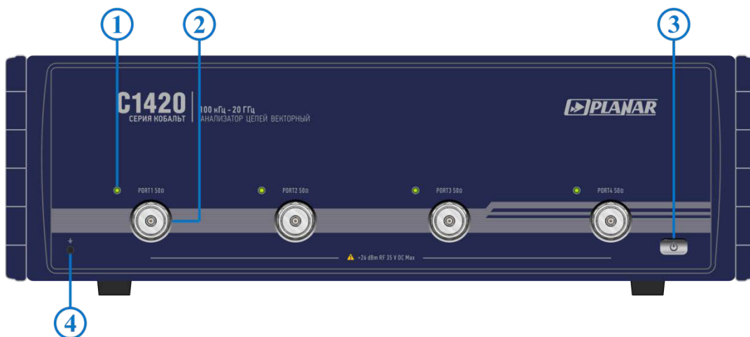
Рисунок 4.13 Передняя панель
