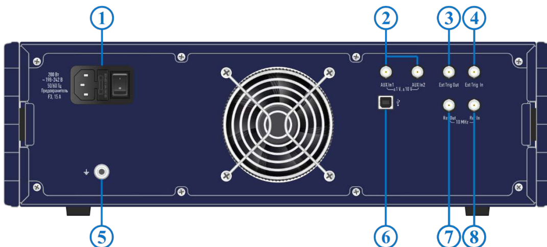
Рисунок 4.14 Задняя панель
