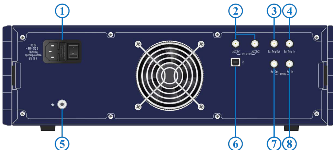
Рисунок 4.20 Задняя панель
