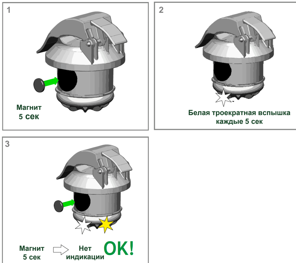
Рисунок 14 – Тестирование индикатора ИКЗ-В51Л
