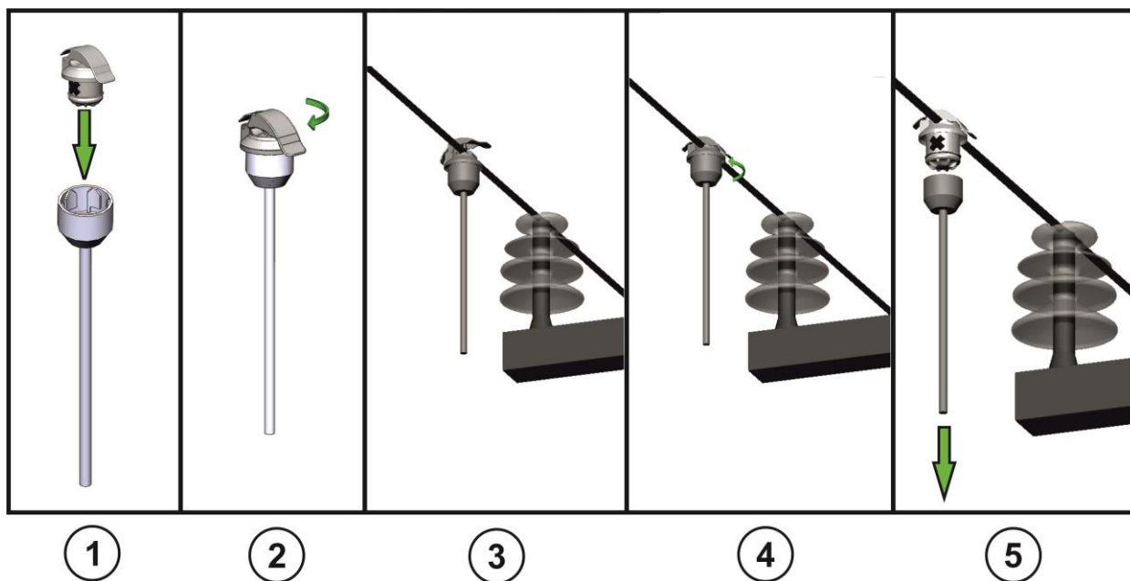
Рисунок 19 – Порядок установки индикатора ИКЗ-В51Л без отключения подачи напряжения
