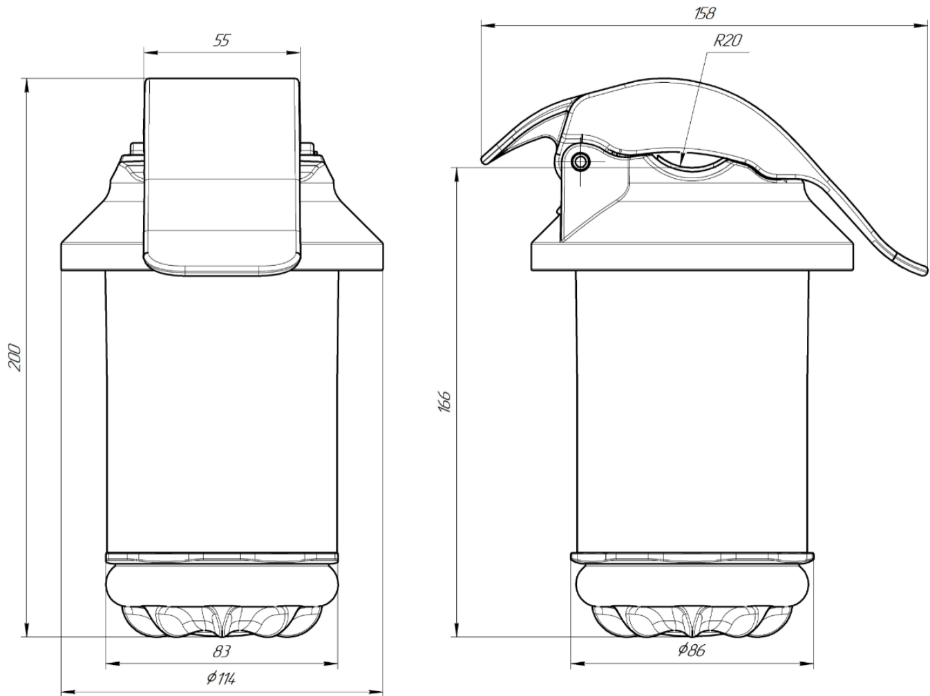
Рисунок 1.1 – Габаритные размеры ИКЗ-В51Л-Master
