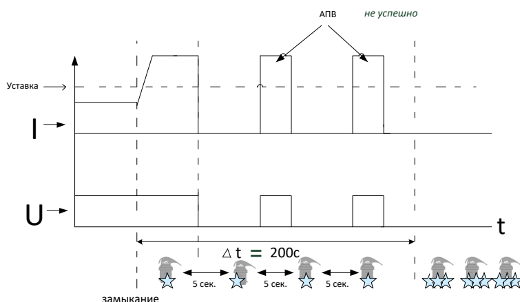
Рисунок 6 – Работа ИКЗ-В51Л при устойчивом замыкании
