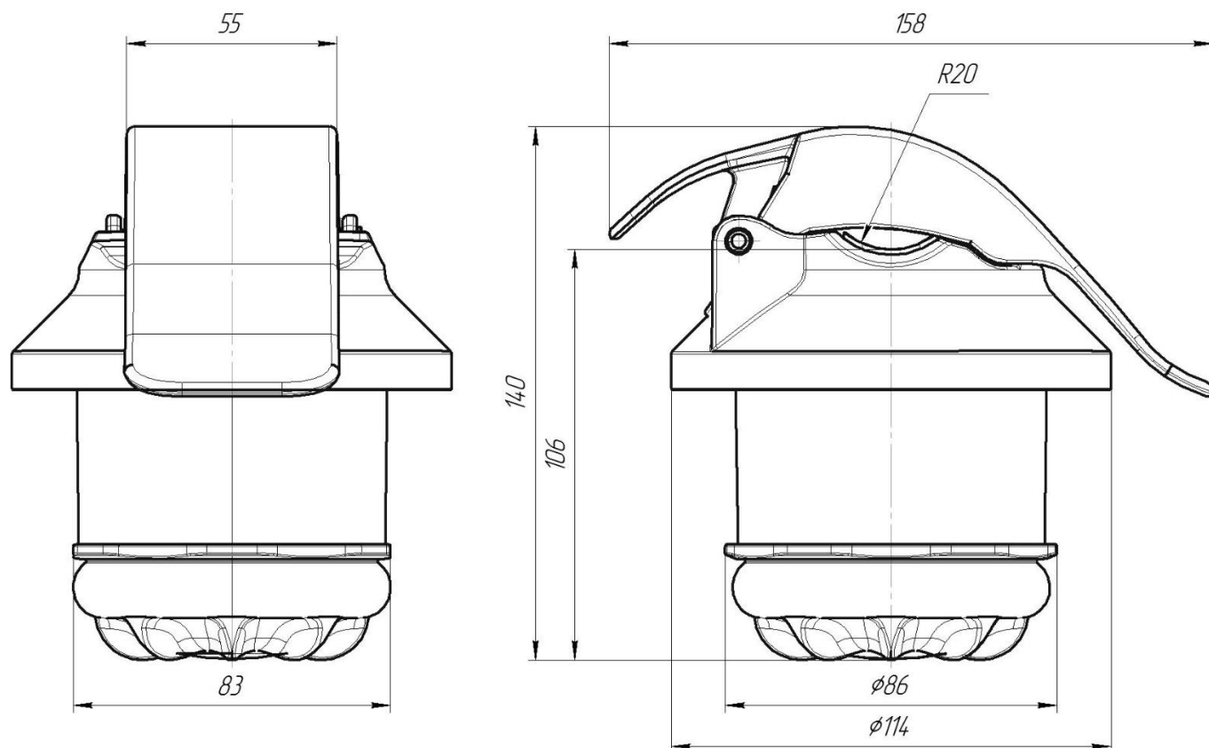
Рисунок 1.1 – Габаритные размеры ИКЗ-В51Л-С
