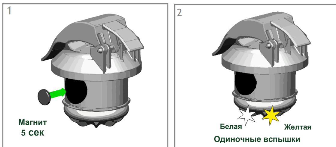
Рисунок 13 – Активация индикатора ИКЗ-В53Л (в первый раз и после изменения настроек)
