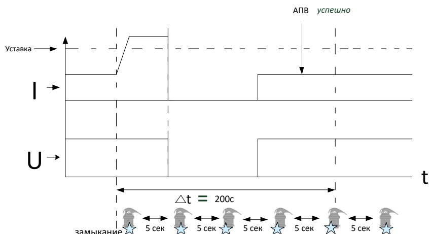
Рисунок 7 – Работа ИКЗ-В51Л при неустойчивом замыкании
