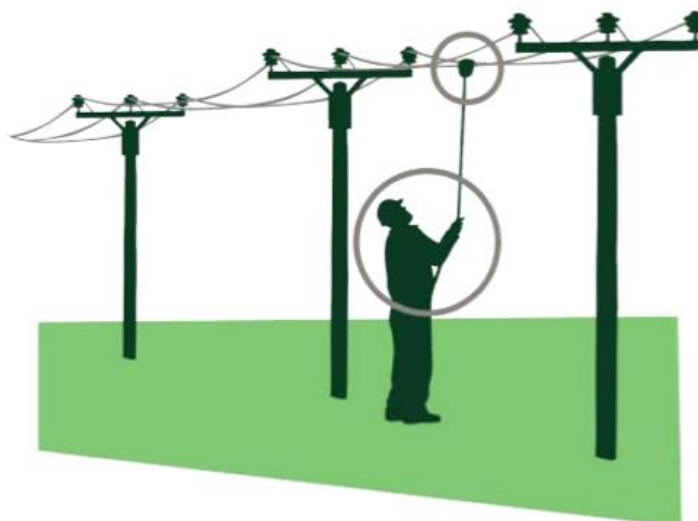
Рисунок 2 – Установка индикатора ИКЗ-В51Л без отключения подачи напряжения
