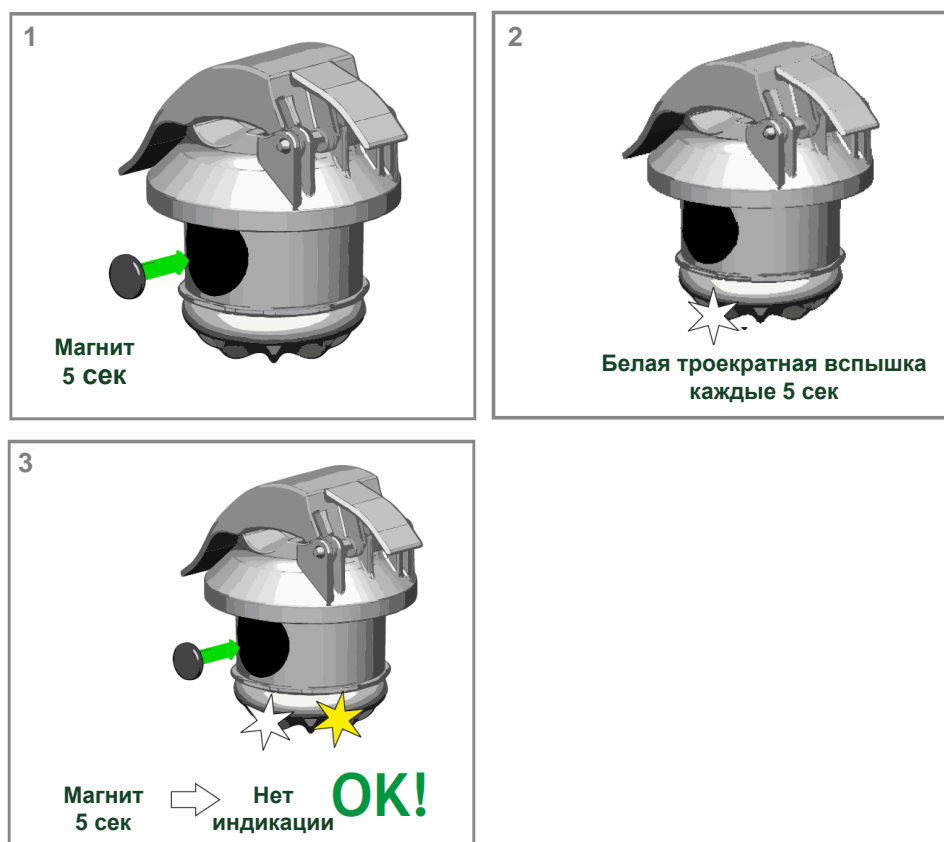
Рисунок 7 – Тестирование индикатора ИКЗ-В53Л-УЗ
