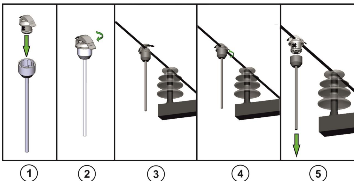
Рисунок 15 – Порядок установки индикатора ИКЗ-В53Л без отключения подачи напряжения
