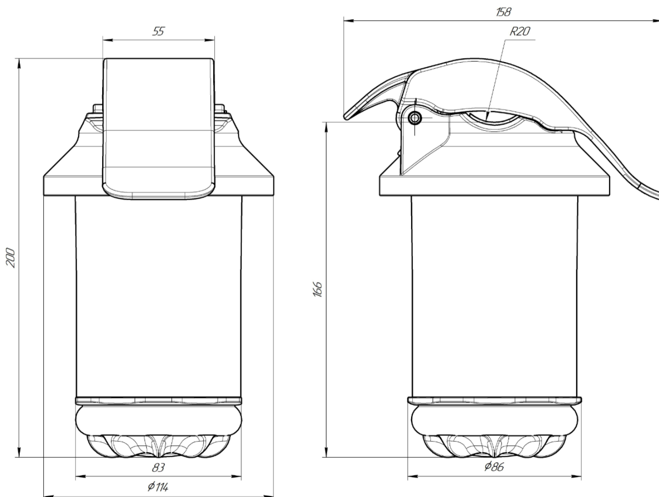
Рисунок 1.1 – Габаритные размеры ИКЗ-В53Л-Master
