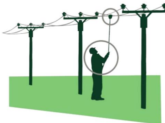
Рисунок 2 – Установка индикатора ИКЗ-В53Л без отключения подачи напряжения
