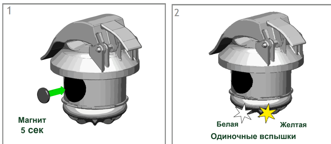
Рисунок 6 – Активация индикатора ИКЗ-В53Л (в первый раз и после изменения настроек)
