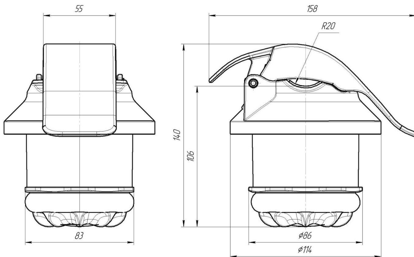
Рисунок 1.2 – Габаритные размеры индикатора ИКЗ-В53Л-С
