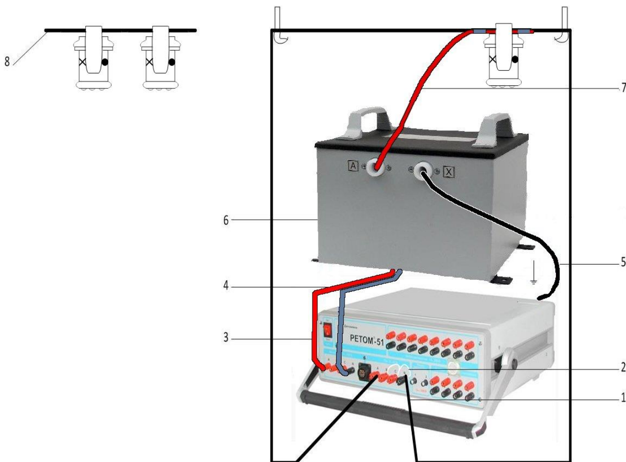
Рисунок 2.3 – Порядок установки
