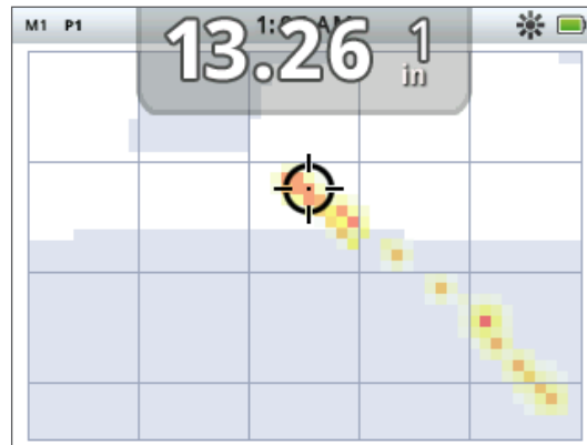
Рисунок 12 – Слежение за целью с показом двух целей (монеты и гвоздя)
