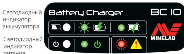
Рисунок 37 – Передняя панель BC 10
