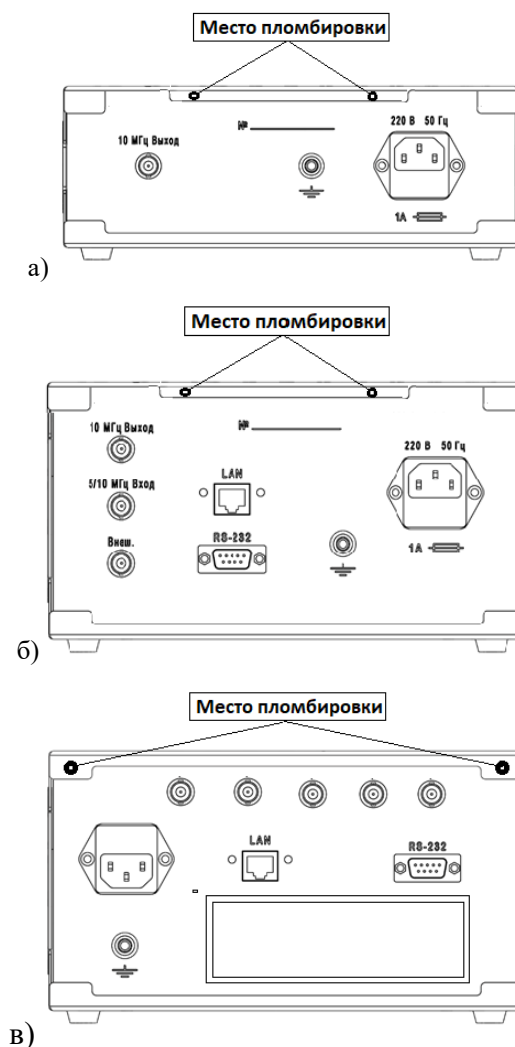
Рисунок 4 – Схема пломбировки от несанкционированного доступа а) ПрофКиП ЧЗ-63, ПрофКиП ЧЗ-84, ПрофКиП ЧЗ-87; б) ПрофКиП ЧЗ-64, ПрофКиП ЧЗ-88, ПрофКиП ЧЗ-96; в) ПрофКиП ЧЗ-99, ПрофКиП ЧЗ-100, ПрофКиП ЧЗ-101, ПрофКиП ЧЗ-102
