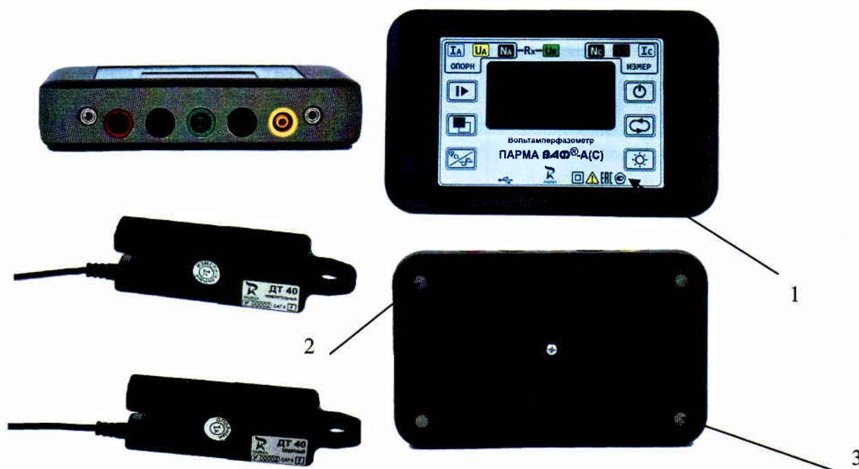
Рисунок 1 – Внешний вид вольтамперфазометра «ПАРМА ВАΦ®-А(С)» с принадлежностями. 1 - знак утверждения типа, 2 – место опломбирования, 3 – место знака поверки.
