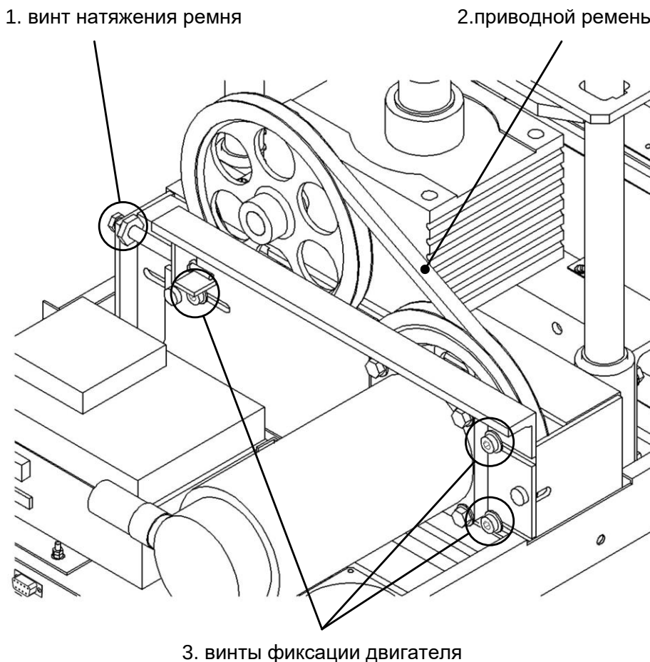
Рисунок 36 – Регулировка натяжения приводного ремня
