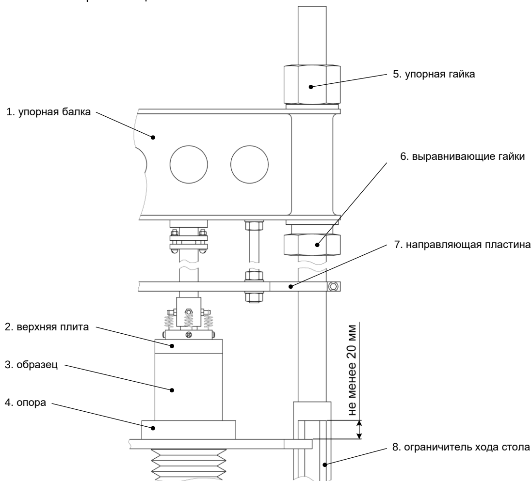
Рисунок 34 – Регулировка положения упорной балки
