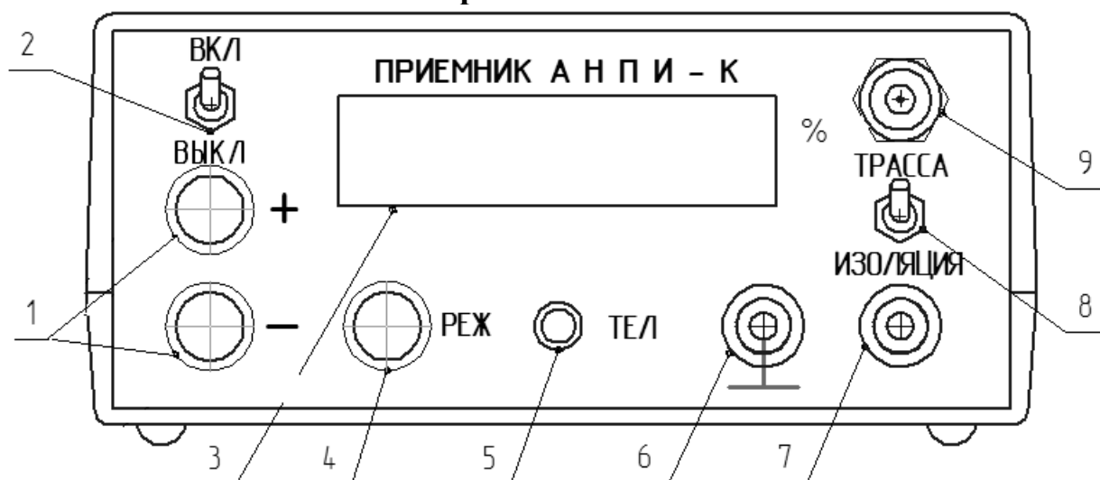
Рис.6. Передняя панель приемника.
