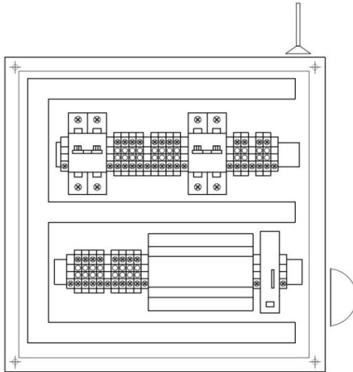
Рисунок 5.1.2 – Расположение оборудования в шкафу Си-Мона
