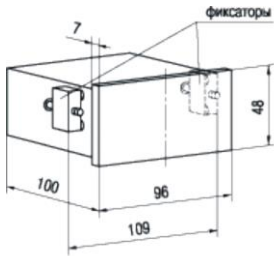
а) щитовое исполнение корпуса
