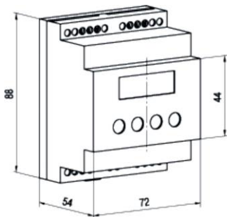
б) исполнение корпуса на DIN-рейку
