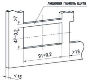
а) щитовое исполнение корпуса
