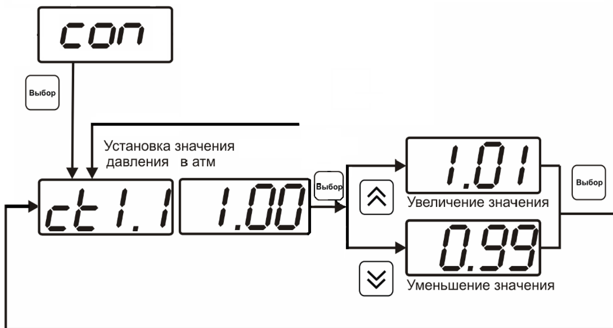
Рисунок 6.12 Задание давления анализируемого газа
