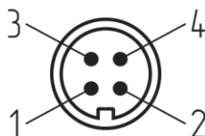
Рисунок 3.3 Разъем подключения измерительного преобразователя
