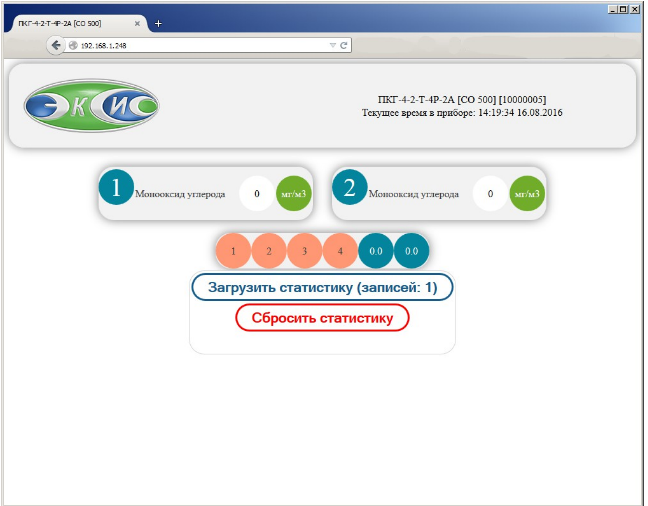
Рисунок 6.43 Web-интерфейс газоанализатора ПКГ-4 /2-Т-К-4Р-2А-Е.
