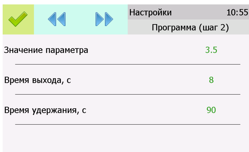
Рисунок 6.32 Вид экрана настройки второго шага программы регулирования
