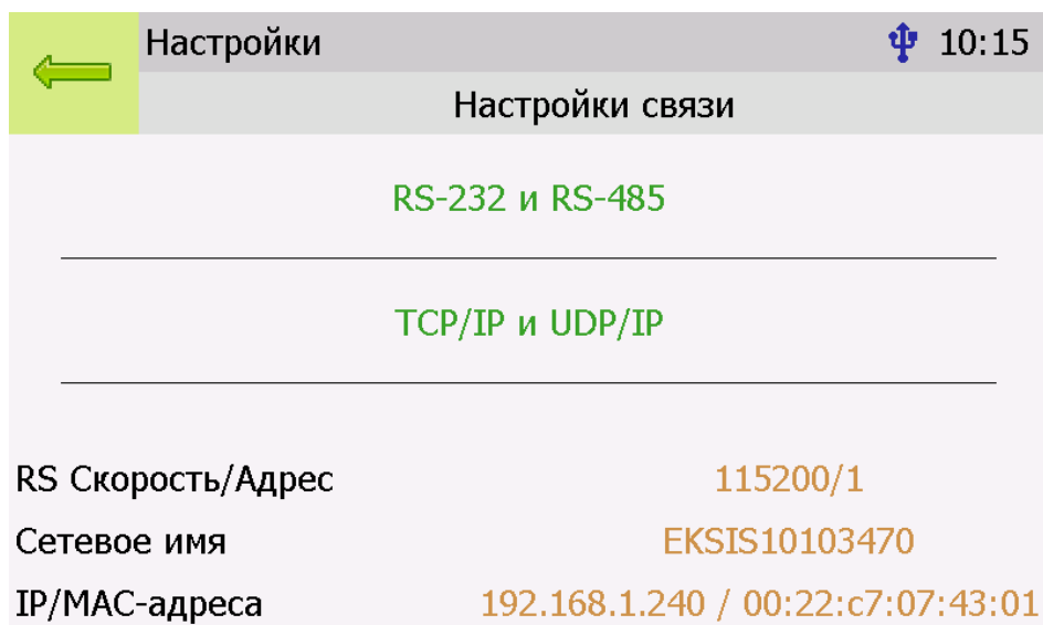
Рисунок 6.37 Экран настроек связи (ПКГ-4 /8-Т-К-УР-ЗА-Е)
