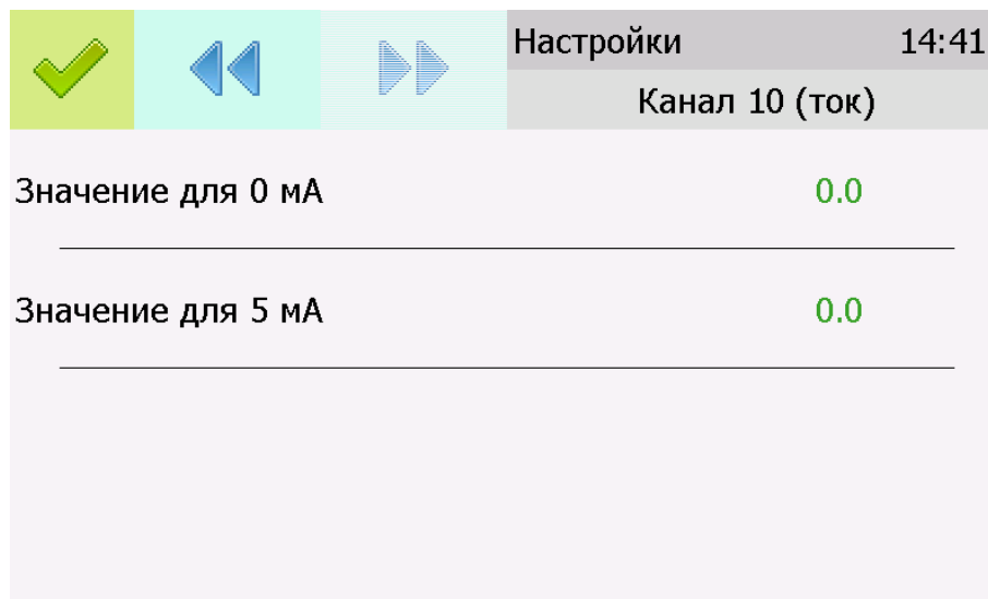
Рисунок 6.35 Вид экрана настройки линейного токового выхода 0...5 мА.
