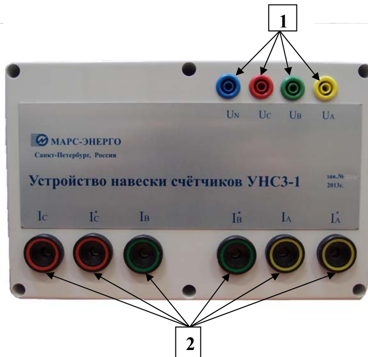
Ри. 3. Блок подключения к установке. 1 – разъемы по напряжению, 2 – разъемы по току
