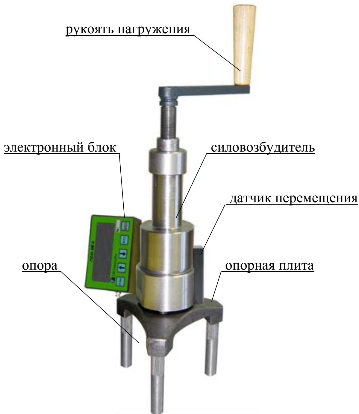
Рисунок 1.а – Общий вид приборов ПСО-5МГ4АД и ПСО-10МГ4АД
