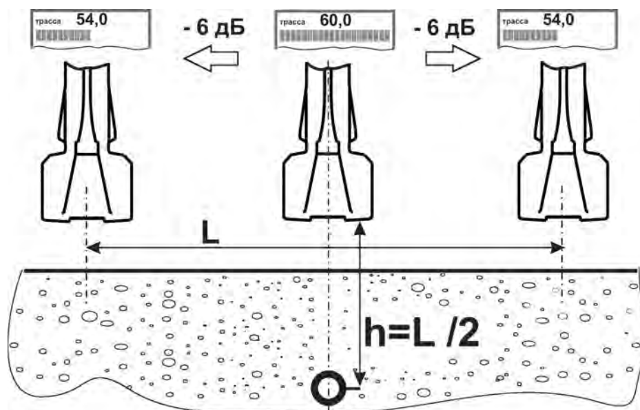
Рисунок 4.3.1 – Определение глубины залегания методом «-6 дБ»
