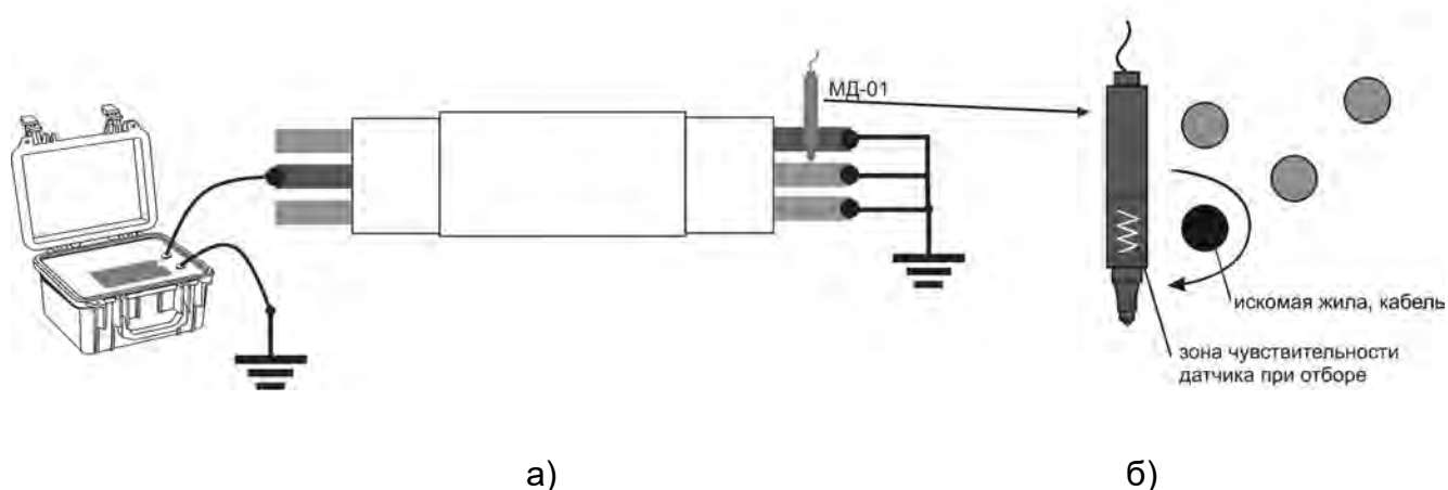
Рисунок 5.4.1 – Схема подключения при отборе жил кабеля
