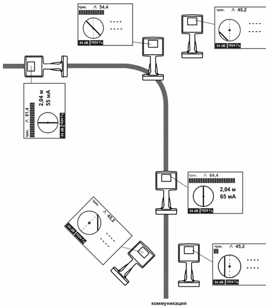
Рисунок 4.2.3 – Поиск с включенной функцией «КОМПАС»
