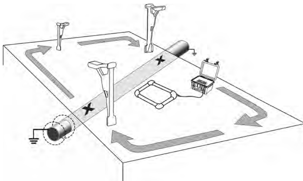
Рисунок 4.4.2.1 – Обследование участков местности с использованием рамки РП-02
