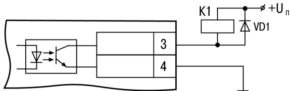
Рисунок 5.8 – Схема подключения нагрузки к ВУ типа K
