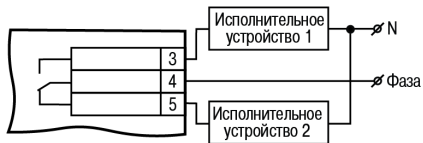
Рисунок 5.7 – Схема подключения нагрузки к ВУ типа P
