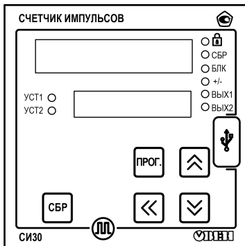
Рисунок 6.2 – Лицевая панель прибора для корпусов настенного И и щитового Щ1 креплений
