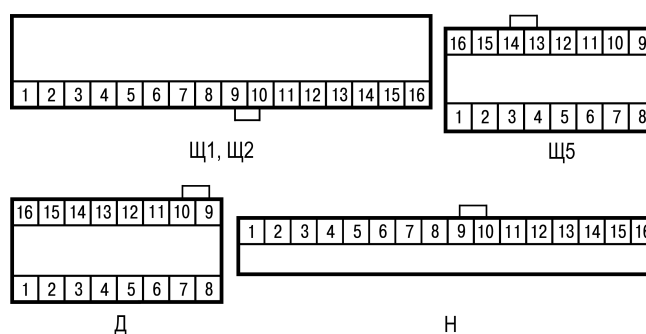
Рисунок 7.7 – Установка переключки
