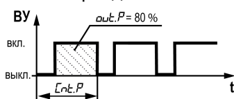
Рисунок 7.4 – Мощность дискретного ВУ
