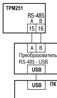
Рисунок 5.15 – Подключение к ПК
