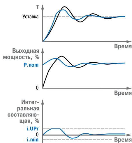
Рисунок 7.9 – Пример ПИД-регулирования 2
