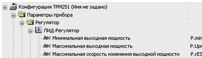
Рисунок 10.10 – Параметры настройки выходной мощности P.Up, P.min и P.rES
