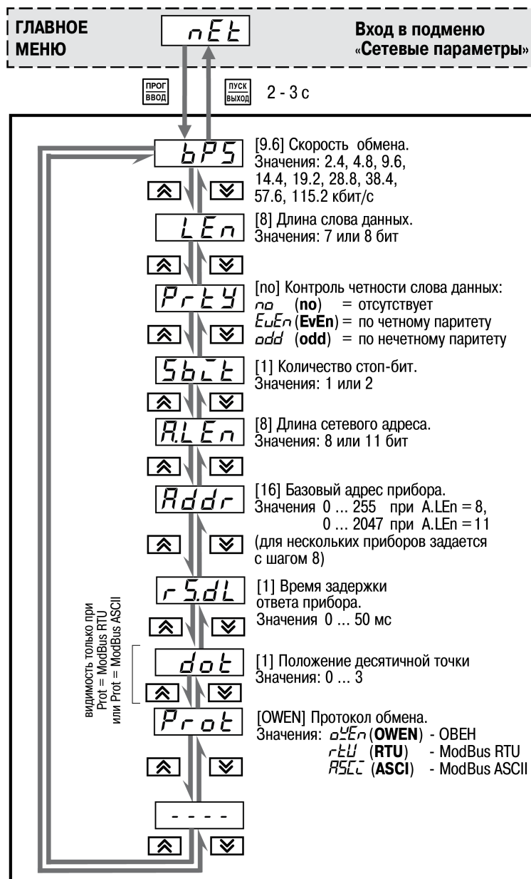
Рисунок 8.9 – Сетевых параметры
