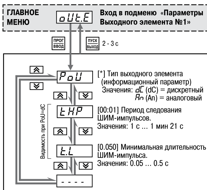
Рисунок 8.7 – Параметры ВЭ1
