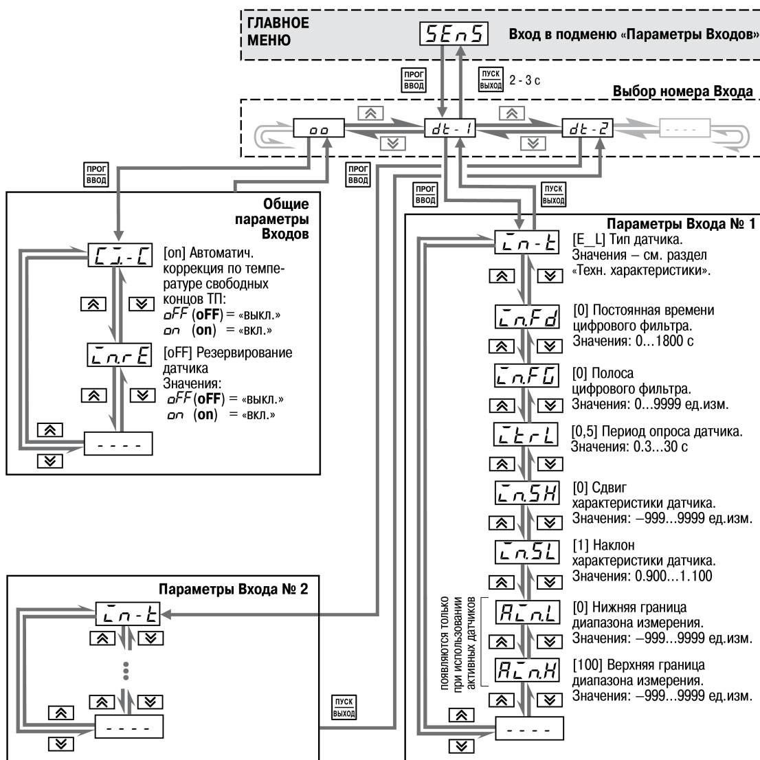
Рисунок 8.6 – Параметры входов
