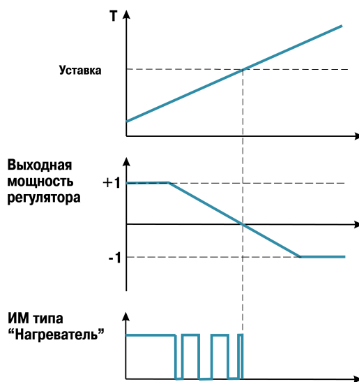
Рисунок 10.9 – Принцип формирования ШИМ-сигнала для «нагревателя»
