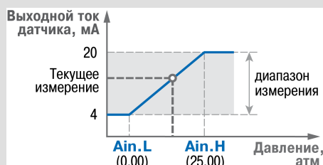
Рисунок 10.6 – Пример задания диапазона измерения
