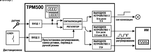
Рисунок 4 – Функциональная схема прибора
