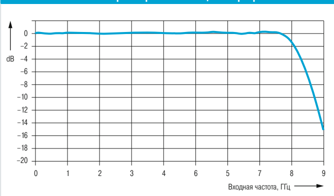
Плоская частотная характеристика осциллографа R&S®RTP084
