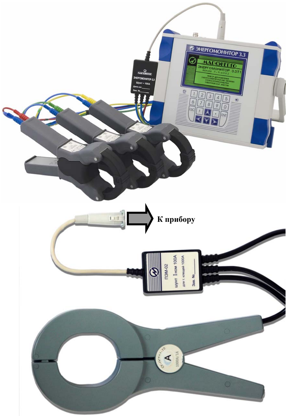
Рис. Б.7. Схемы подключения токоизмерительных клещей 1000 А к Прибору ЭМ-3.3Т1 через Шунт 100 А
