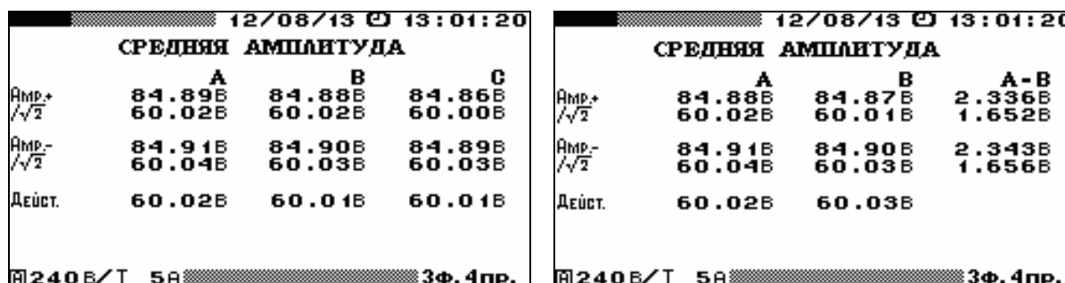
Рис. 4.58. Отображение амплитудных значений напряжения в режиме «СРЕДНЯЯ АМПЛИТУДА»
