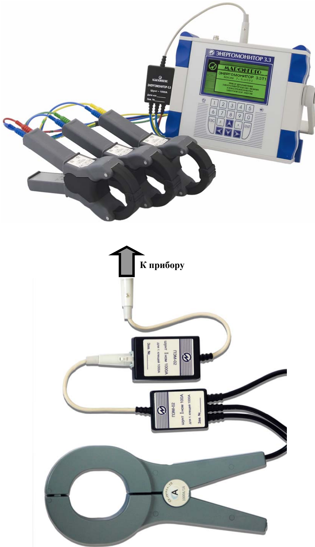
Рис. Б.6. Схемы подключения токоизмерительных клещей 1000 А к Прибору ЭМ-3.3Т1 через Шунт 1000 А
