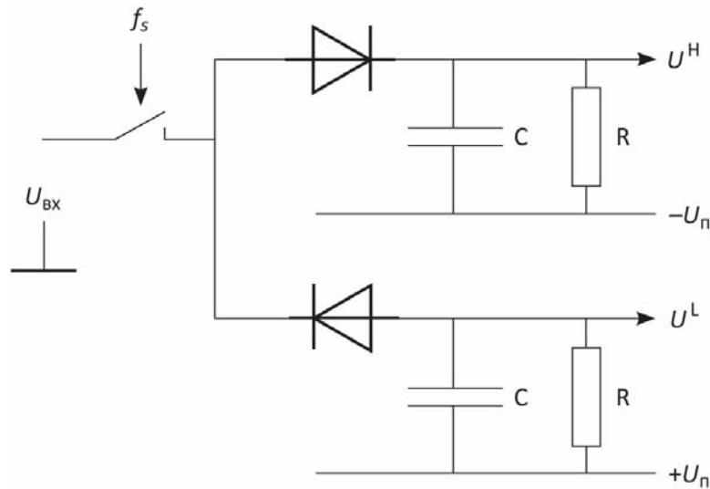
Рис. 4.53. Принцип обработки входного сигнала в режиме «АМПЛИТУДНЫЙ ДЕТЕКТОР»: U_{вх} — входное напряжение; f_s — частота дискретизации (12,8 кГц); U^H — значения огибающей напряжения сверху; U^L — значения огибающей напряжения снизу; \tau = RC — постоянная времени (задается в диапазоне от 0,1 до 100 с); -U_{п} — минимально возможное напряжение; +U_{п} — максимально возможное напряжение
