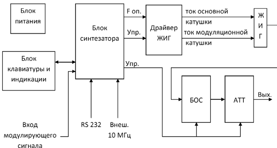
Рис 5.1 Структурная схема генератора
