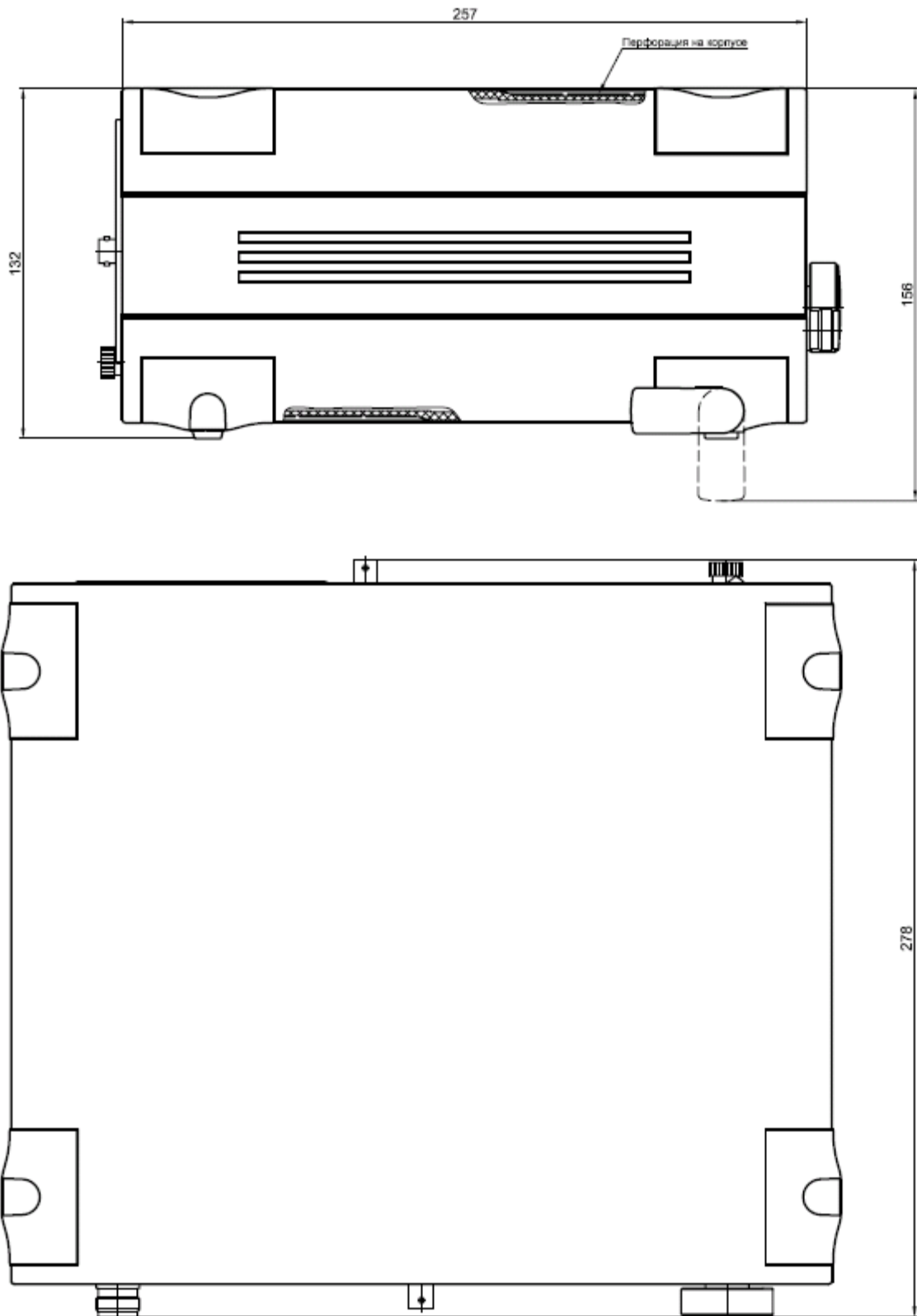
Общий вид генератора Г4-225 и его габаритные размеры
