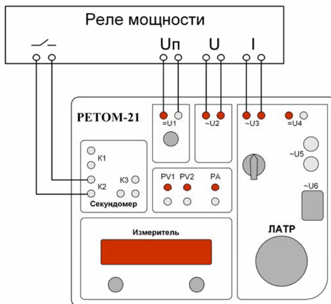
Рисунок 14.3 – Схема подключения реле мощности
