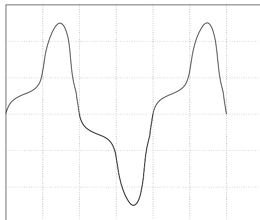
Рисунок 8.7 – Кривая потребления тока персонального компьютера
