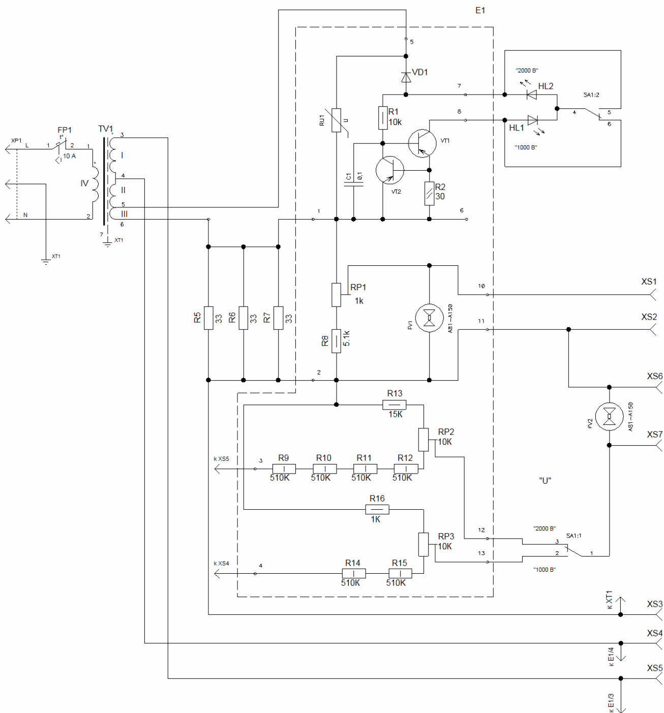
Рисунок Д.2 - Схема электрическая принципиальная блока PET-BAX-2000
