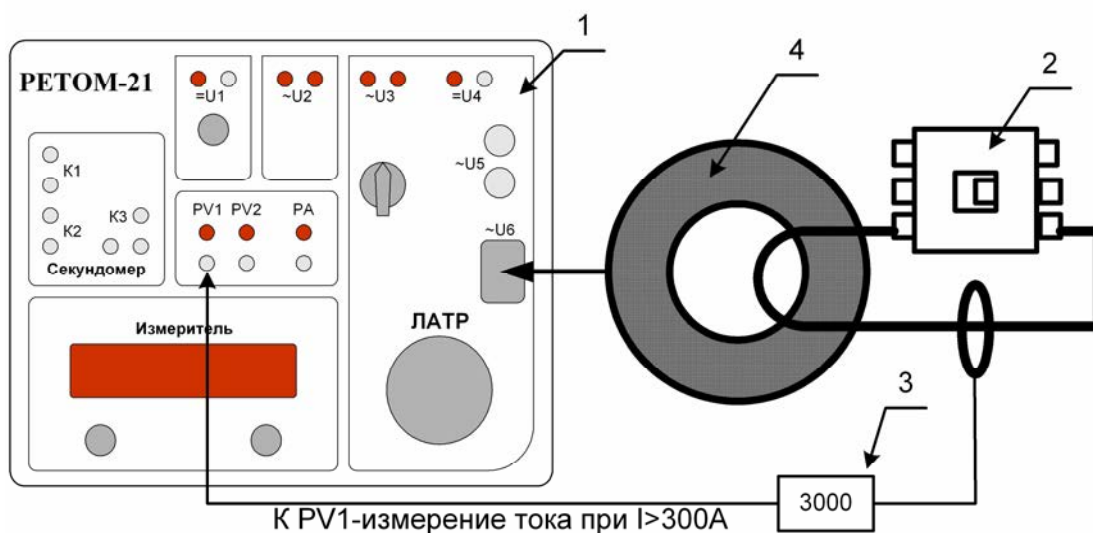
Рисунок 14.14 – Проверка выключателей с помощью РЕТОМ-21 и РЕТ-3000 в режиме фиксации от измерителя PV1 (по току)
