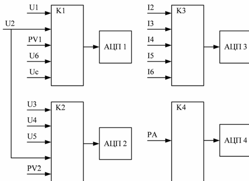
Рисунок 8.1 – Функциональная схема мультиметра
