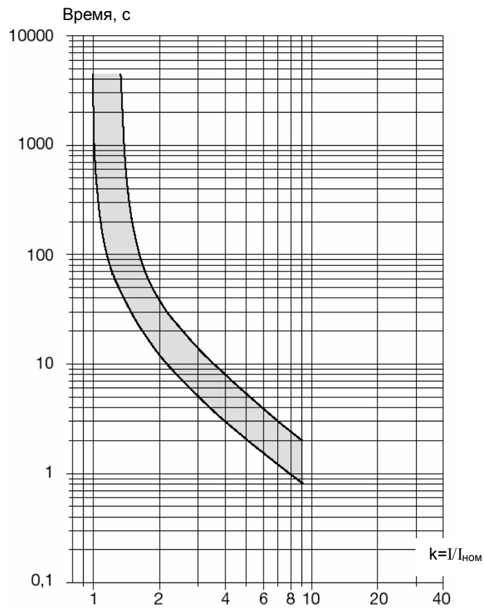
Рисунок 5.2 – Зависимость времени срабатывания термореле от выходного тока
