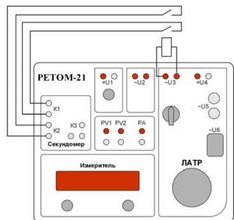
Рисунок 9.7 – Схема подключения для измерения разновременности срабатывания и возврата
