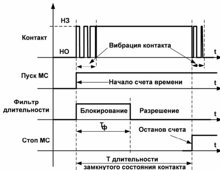
Рисунок 9.3 – Диаграмма измерения длительности кратковременного переключения контакта
