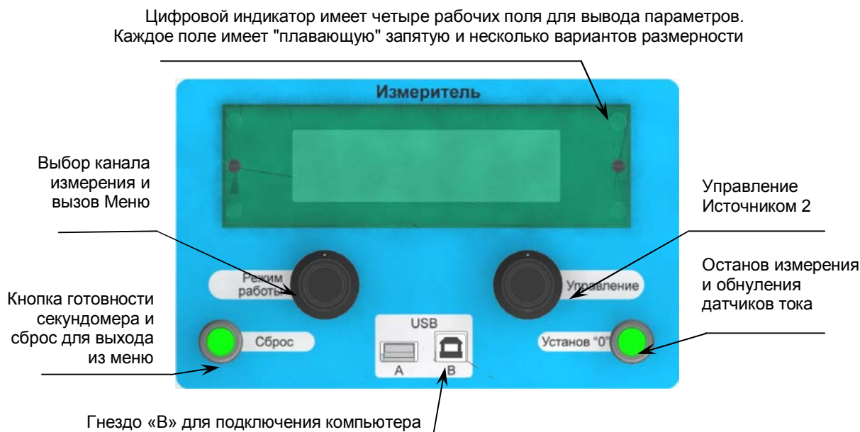
Рисунок 7.1 – Функциональные элементы пульта управления
