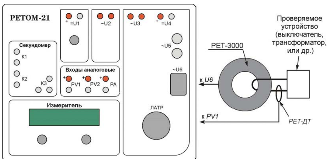
Рисунок 12.3 – Схема проверки различного электрооборудования с помощью РЕТ-3000
