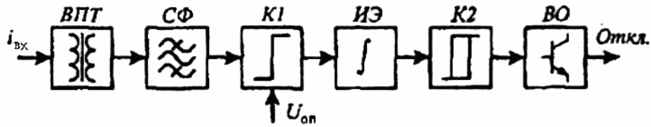
Рисунок 14.5 – Структура реле РТЗ-51
