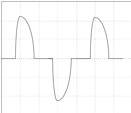
Рисунок 8.6 – Кривая потребления тока нелинейной нагрузки
