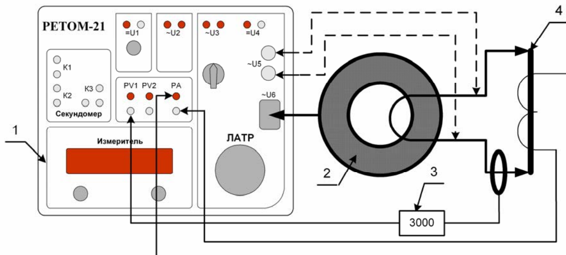
Рисунок 14.17 – Схема проверки полярности и коэффициента трансформации ТТ с применением блока РЕТ-3000
