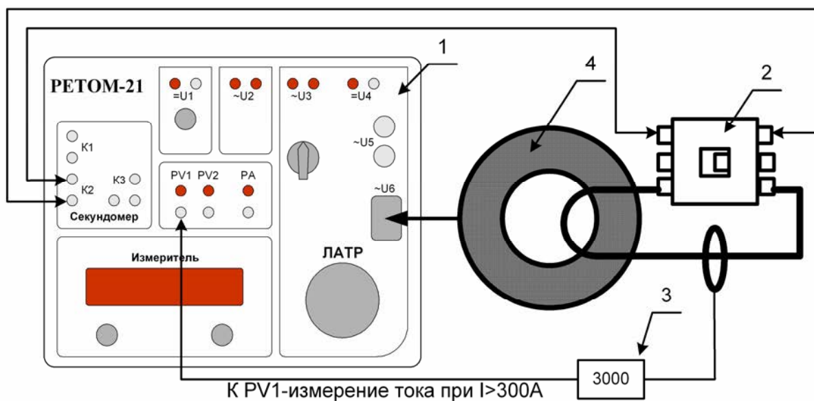
Рисунок 14.15 – Проверка выключателей с помощью РЕТОМ-21 и РЕТ-3000 в режиме фиксации от секундомера (по контакту)
