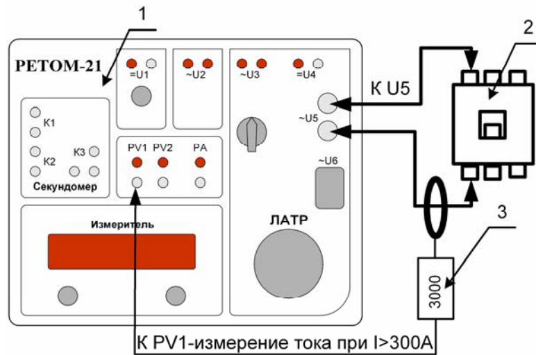
Рисунок 14.12 – Проверка выключателей с помощью РЕТОМ-21 в режиме фиксации по току от измерителя PV1
