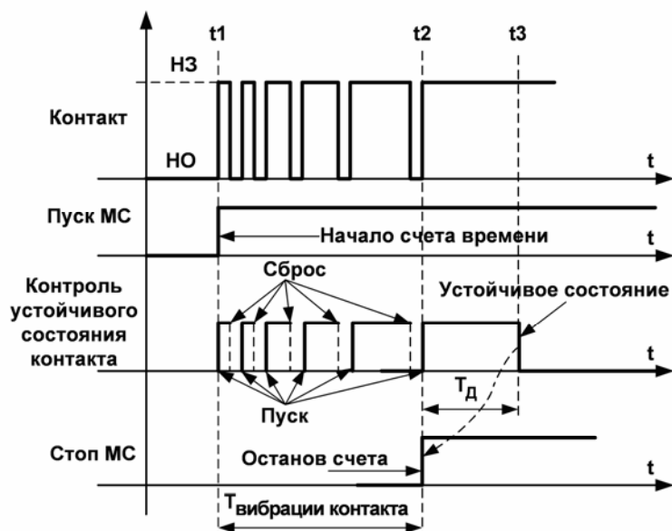
Рисунок 9.4 – Диаграмма измерения времени дребезга контакта
