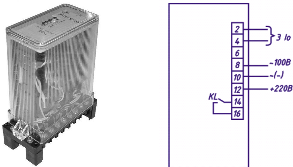
Рисунок 14.4 – Реле РТЗ-51
