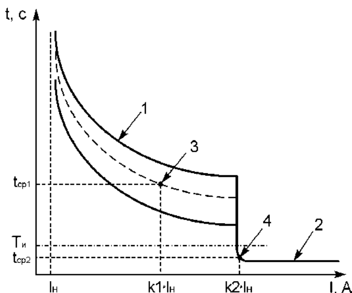
Рисунок 14.11 – Времятоковая характеристика автоматического выключателя
