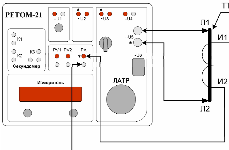
Рисунок 14.16 – Схема проверки полярности и коэффициента трансформации ТТ
