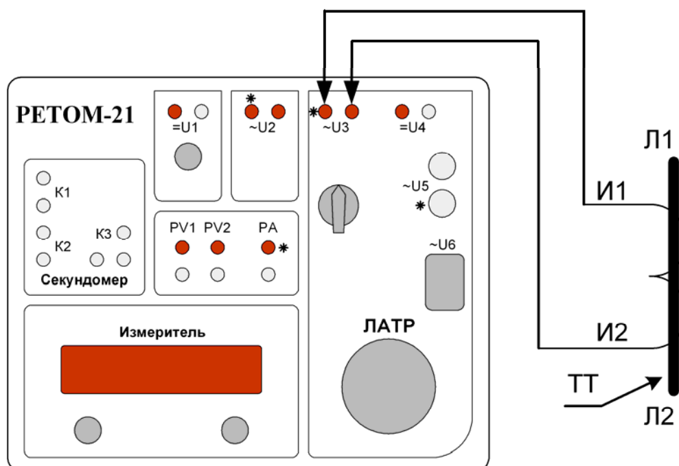
Рисунок 14.18 – Схема измерения характеристики намагничивания ТТ
