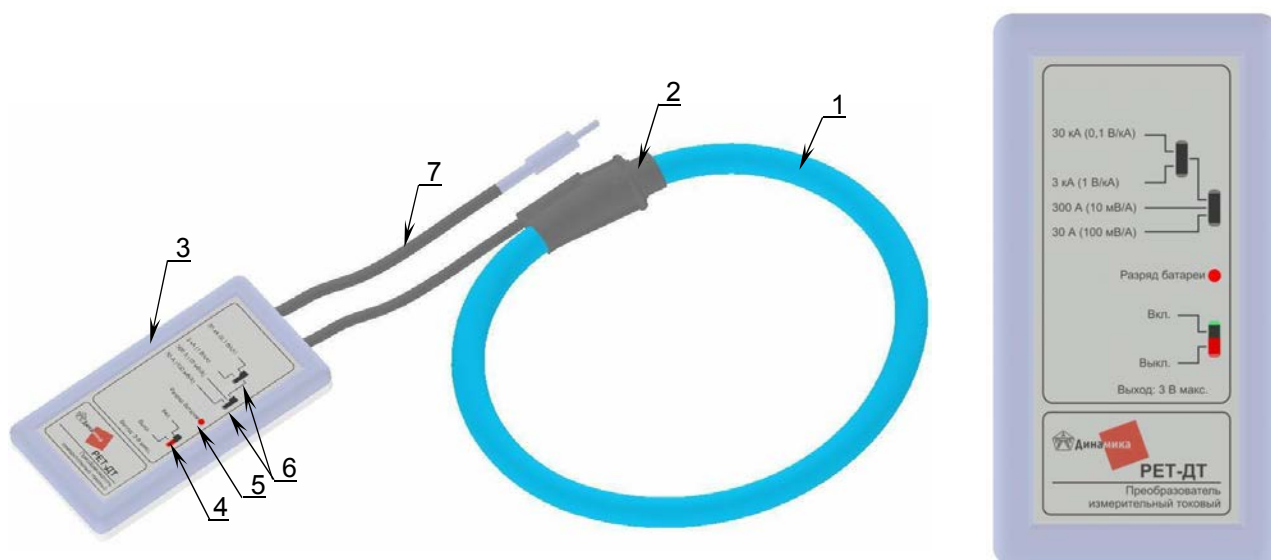
1 - измерительное кольцо; 2 - байонетный замок; 3 - интегратор; 4 - включение; 5 - индикатор разряда батареи; 6 - выбор диапазона; 7 - выходной кабель
