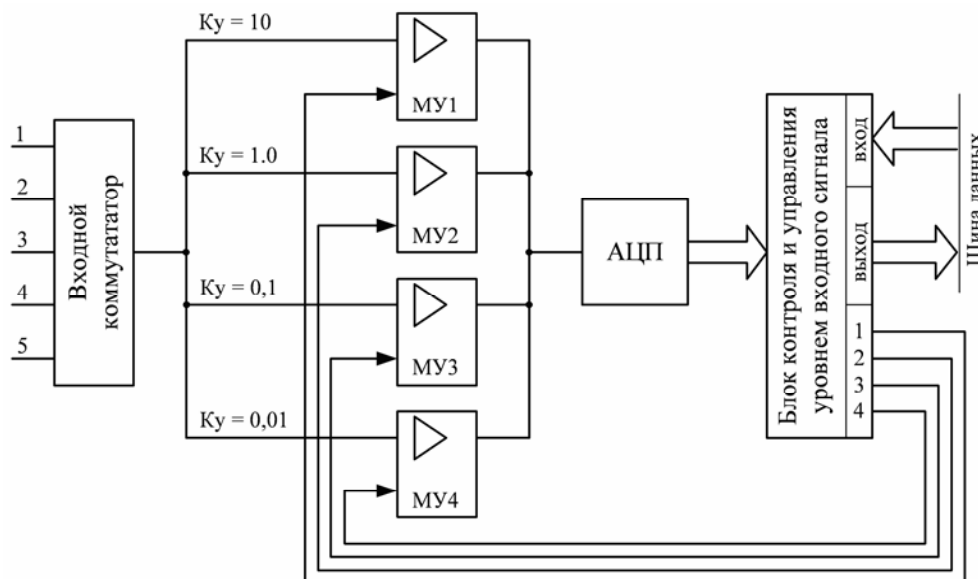
Рисунок 8.2 – Переключаемый четырехуровневый масштабный усилитель
