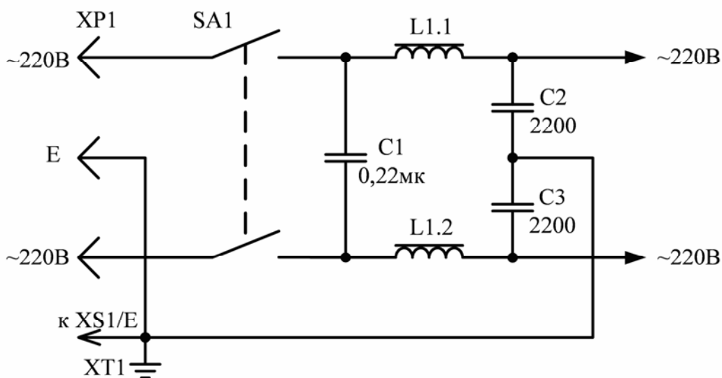
Рисунок 6.2 – Электрическая схема входной части устройства
