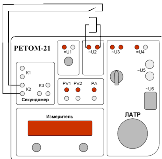
Рисунок 14.1 – Схема подключения реле напряжения
