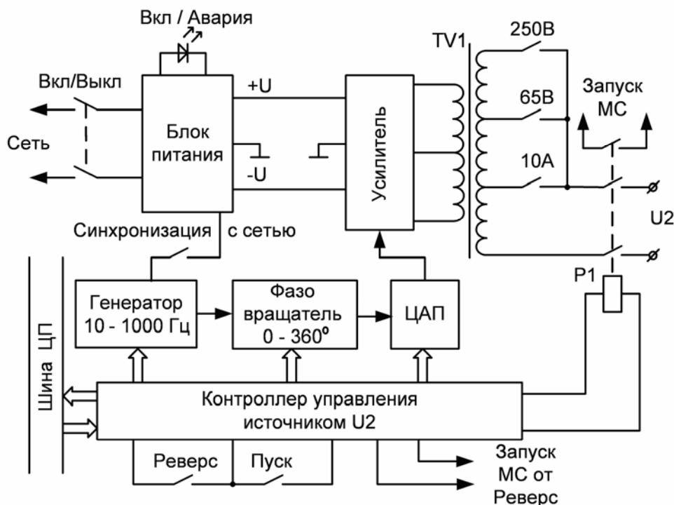
Рисунок 11.2 – Функциональная схема Источника 2
