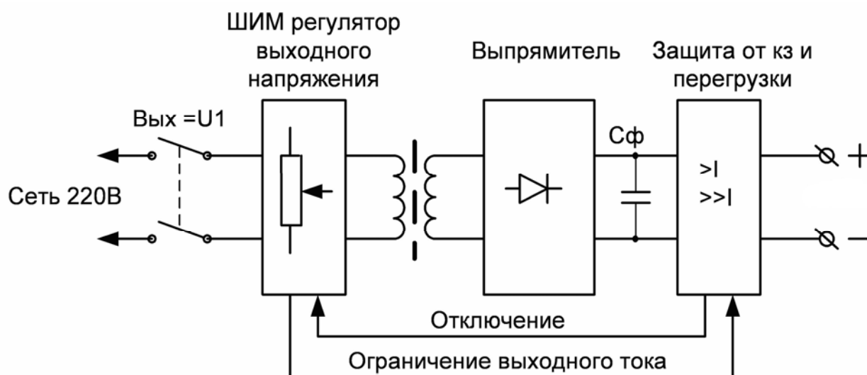
Рисунок 10.2 – Функциональная схема Источника 1
