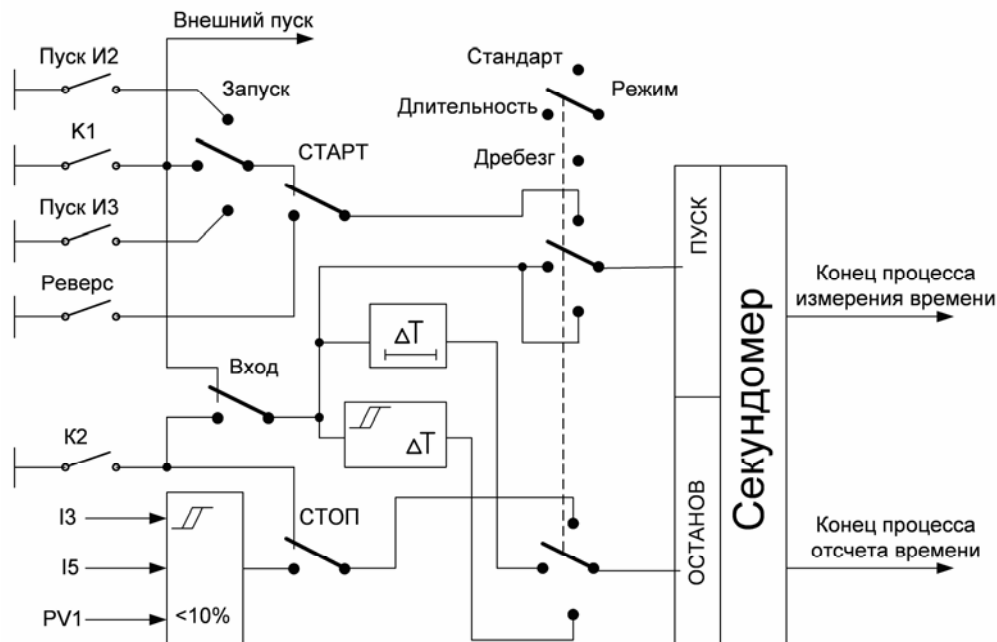
Рисунок 9.2 – Логическая схема работы секундомера
