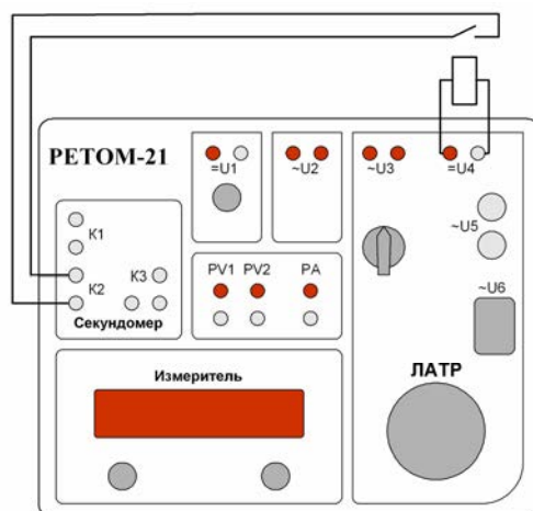
Рисунок 14.2 – Схема подключения промежуточного реле
