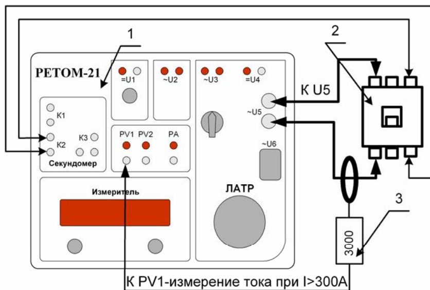
Рисунок 14.13 – Проверка выключателей с помощью РЕТОМ-21 в режиме фиксации по контакту
