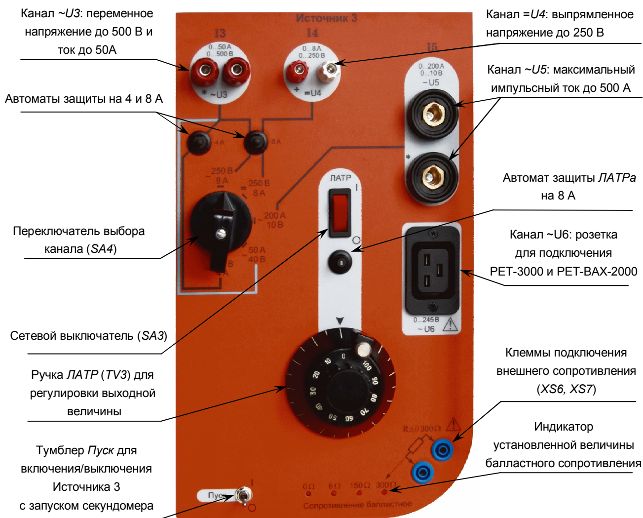
Рисунок 12.1 – Функциональные элементы Источника 3
