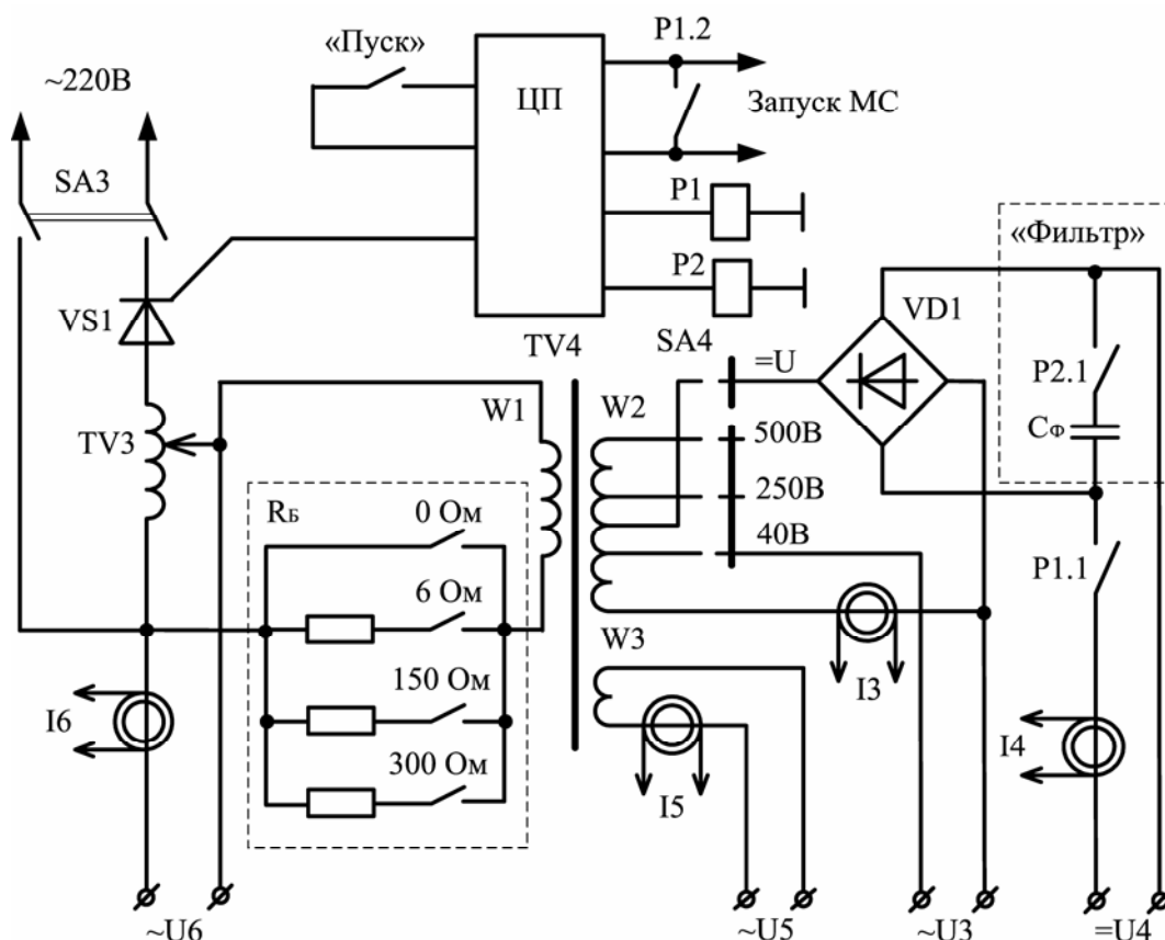
Рисунок 12.2 – Функциональная схема Источника 3
