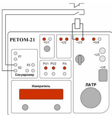
Рисунок 9.6 – Схема подключения для измерения времени срабатывания и возврата
