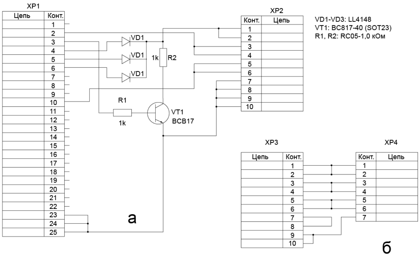
Схемы кабеля: «LPT – разъем» (а), «шлейф – разъем (к прибору)» (б)
