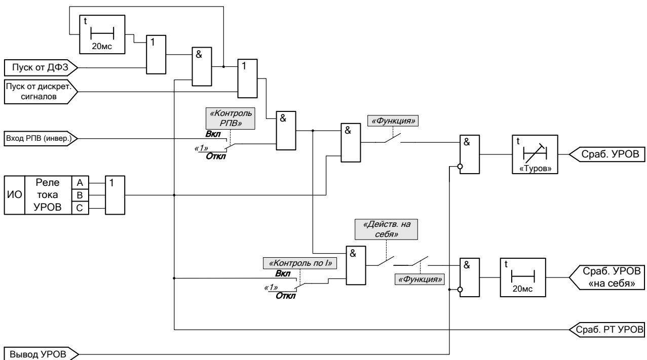
Рисунок 17 – Функционально-логическая схема блока УРОВ
