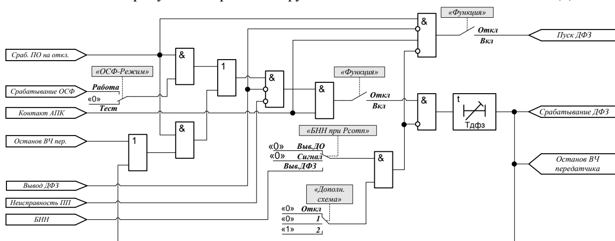
Рисунок 16 – Функционально-логическая схема блока ДФЗ
