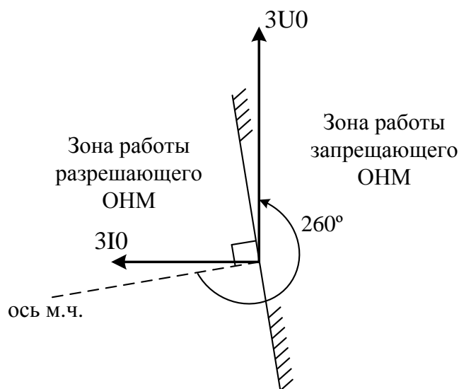
Рисунок 7 – Векторная диаграмма, поясняющая работу ОММ НП-р (отсчет идет от линии м.ч. до фиксированной оси напряжения; положительное направление – против направления вращения часовой стрелки)
