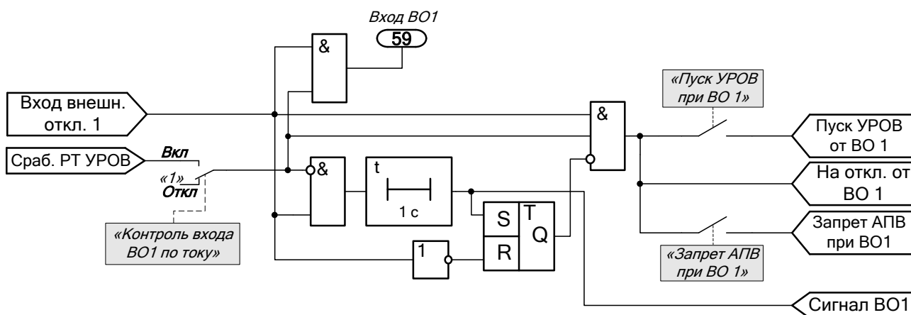
Рисунок 15 – Функционально-логическая схема блока отключения выключателя от сигнала внешнего отключения 1
