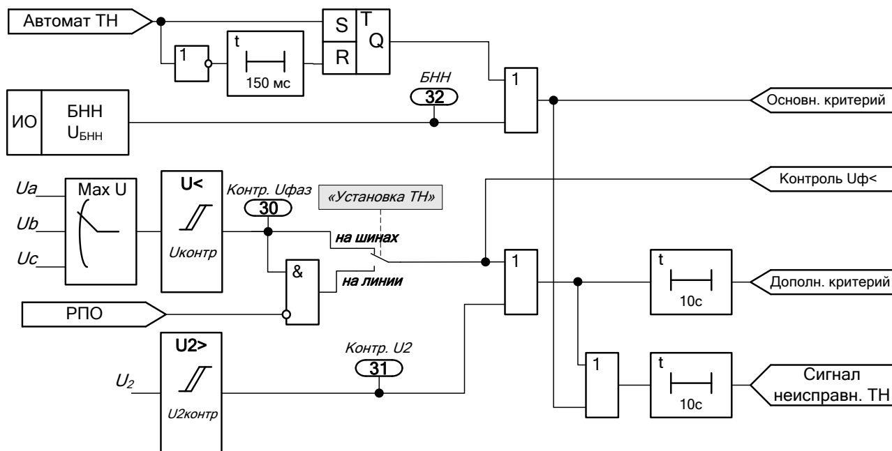
Рисунок 1 – Функционально-логическая схема блока выявления неисправностей в цепях ТН
