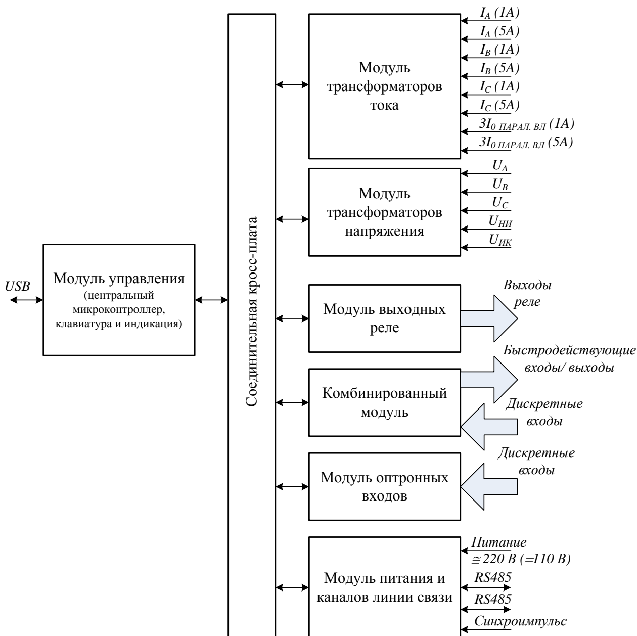
Рисунок 20 – Структурная схема устройства «Сирius-3-ДФ3-01»
