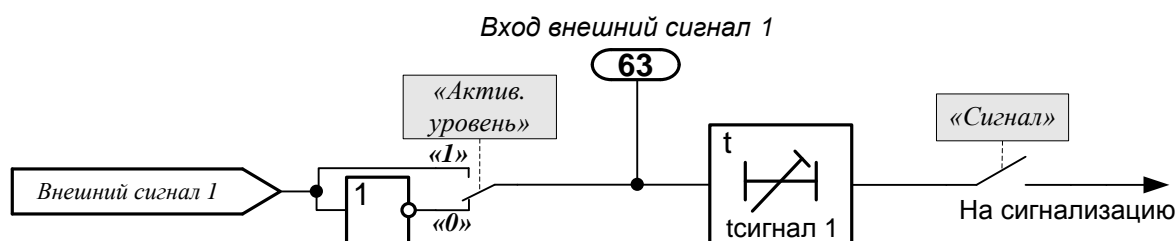
Рисунок 16 – Схема реализации входа «Внешний сигнал 1»
