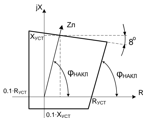
Рисунок 5 – Характеристика срабатывания ИО РС
