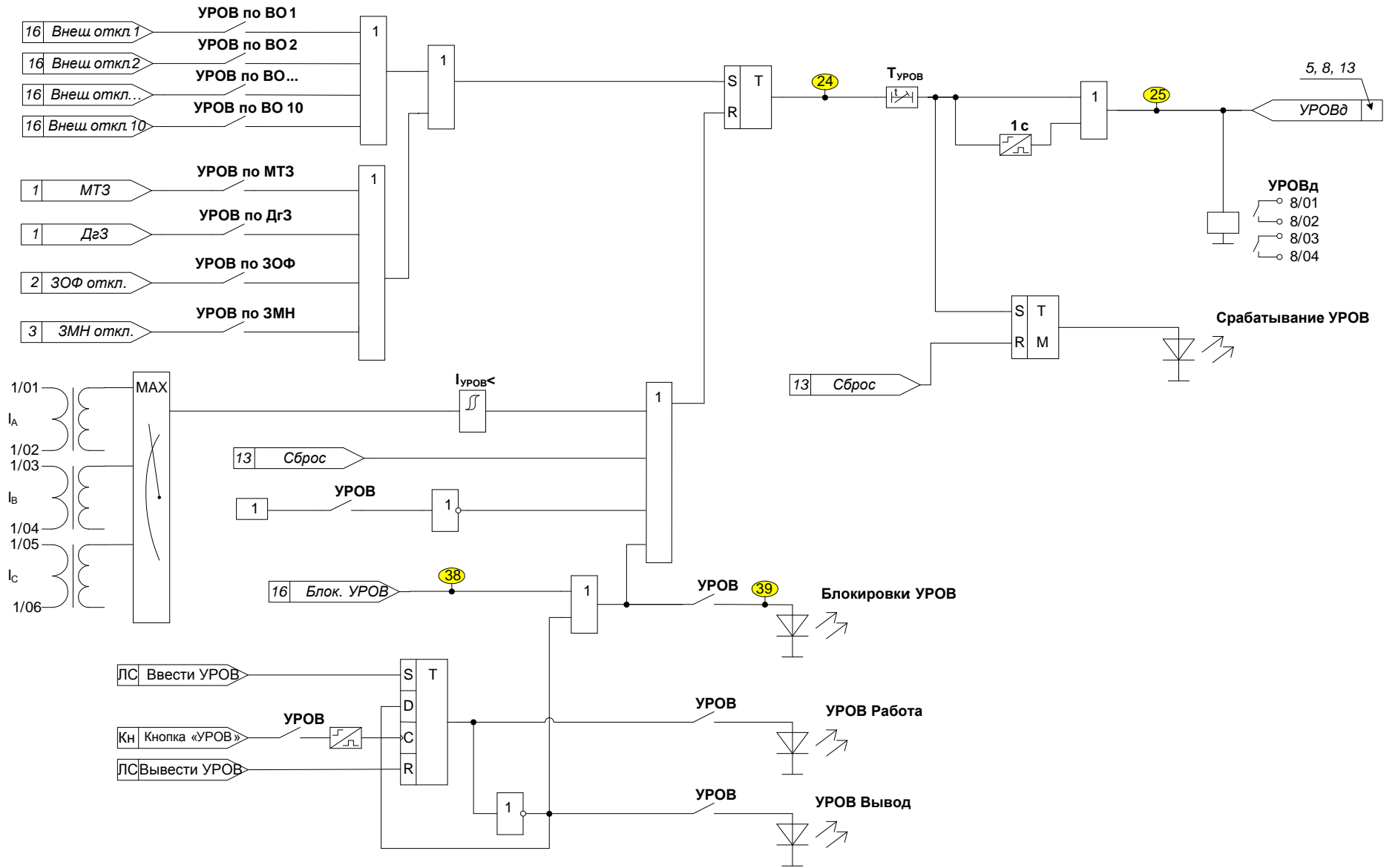
Рисунок Д.6 – Функциональная схема алгоритма УРОВ
