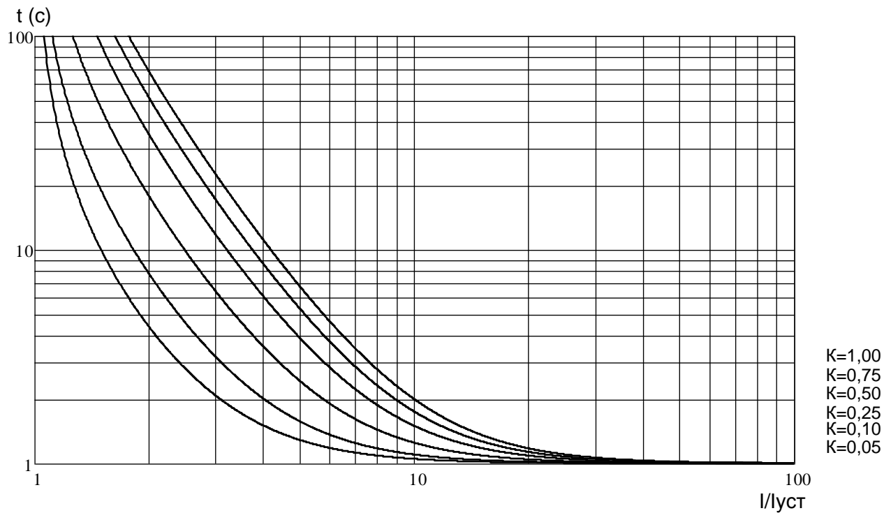
Рисунок Е.5 – Ультра инверсная характеристика по МЭК 255-4
