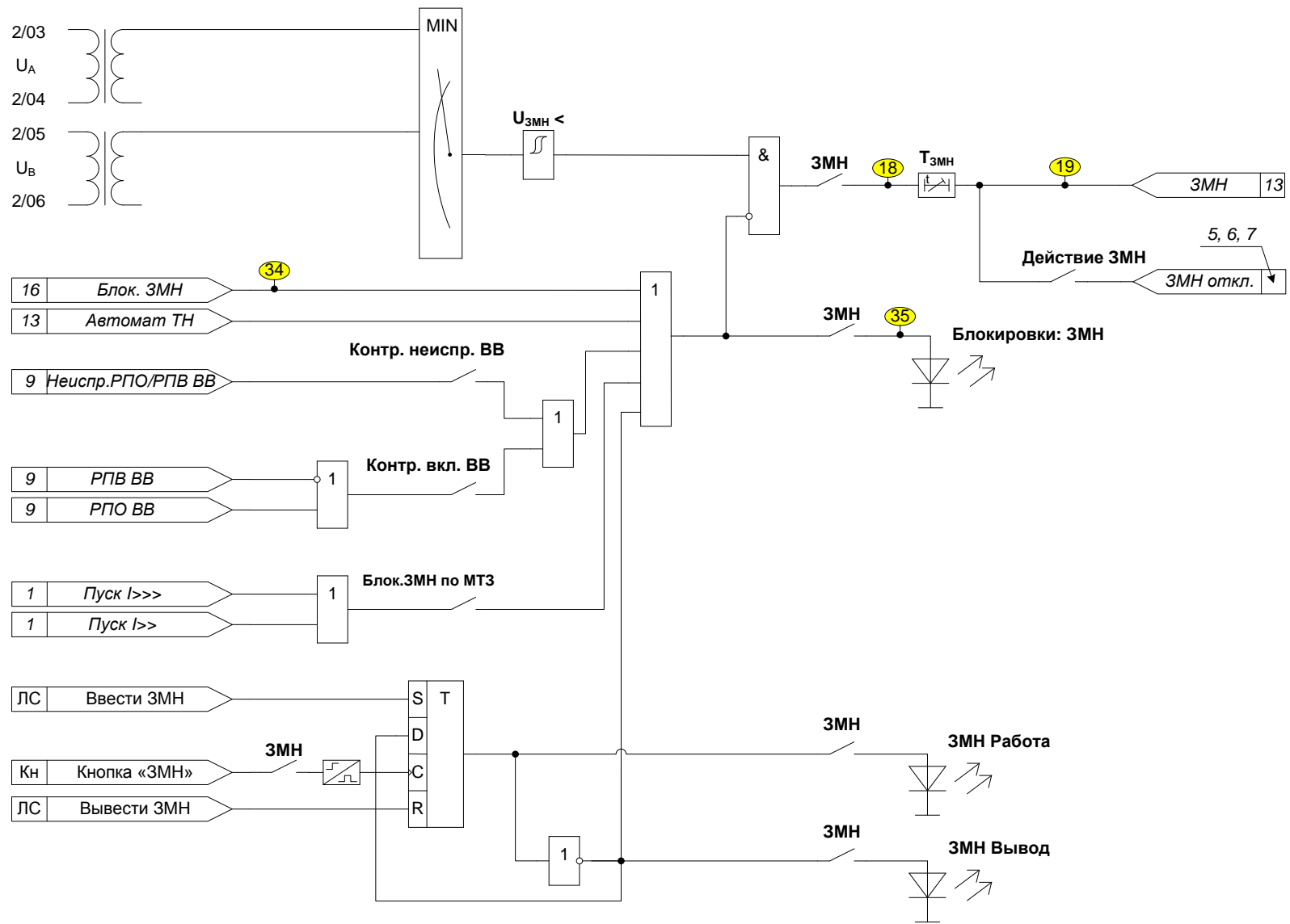
Рисунок Д.3 – Функциональная схема алгоритма ЗМН
