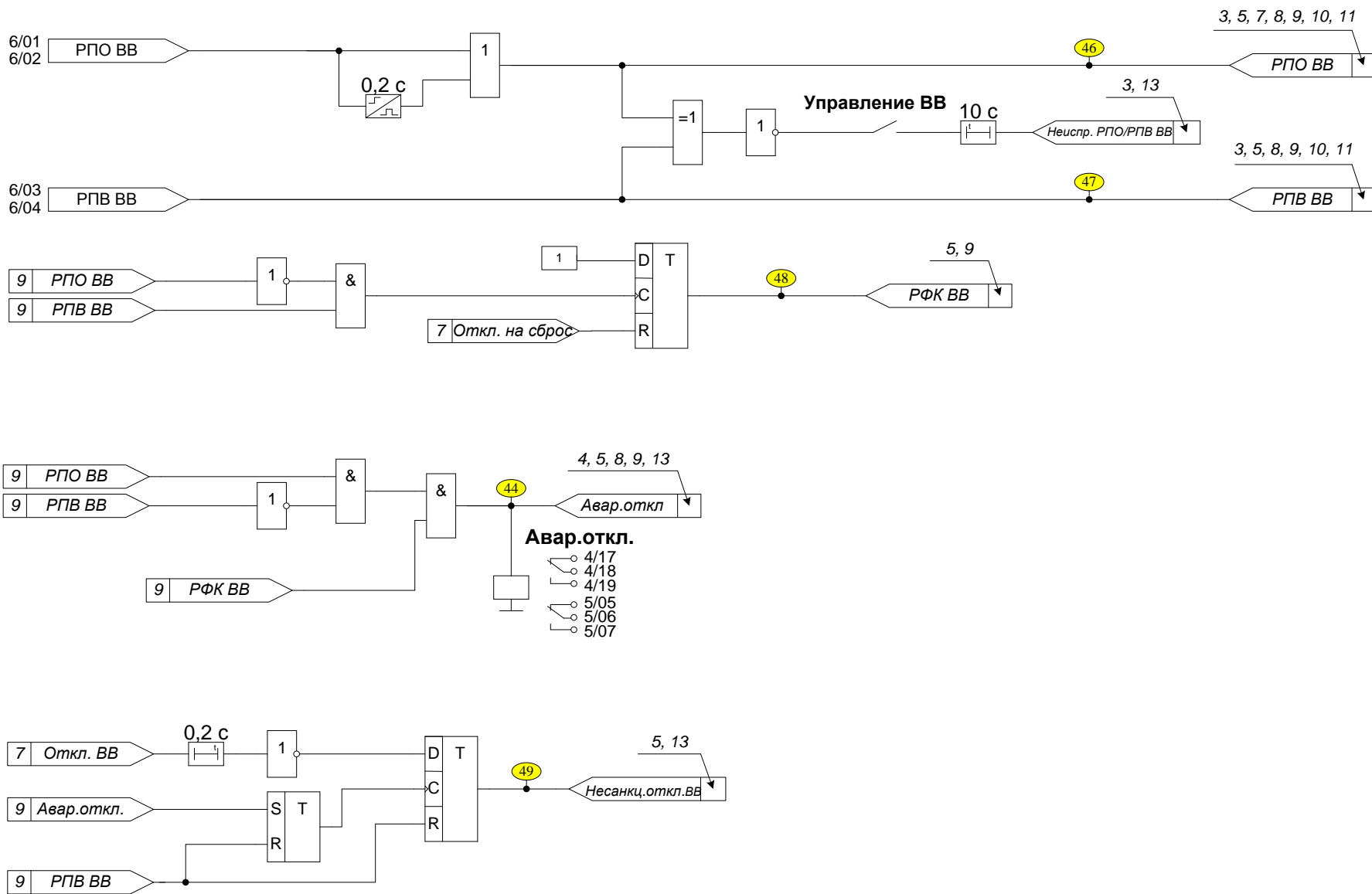
Рисунок Д.9 – Функциональная схема алгоритма диагностики ВВ
