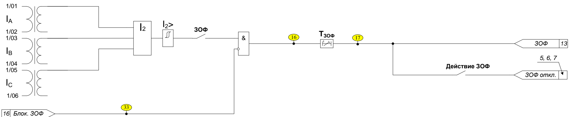
Рисунок Д.2 – Функциональная схема алгоритма ЗОФ
