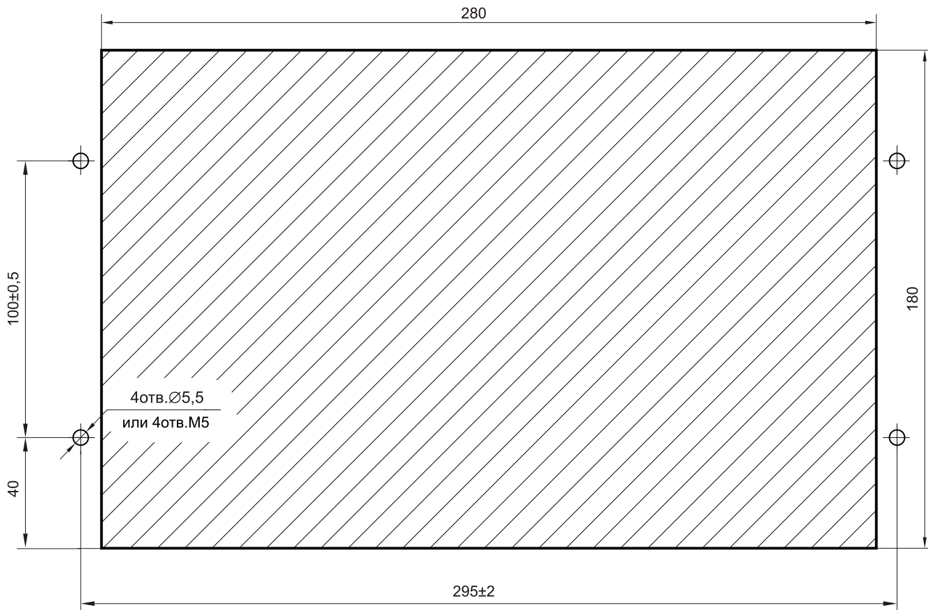
Рисунок В.5 – Разметка панели под установку устройства (установочные размеры)
