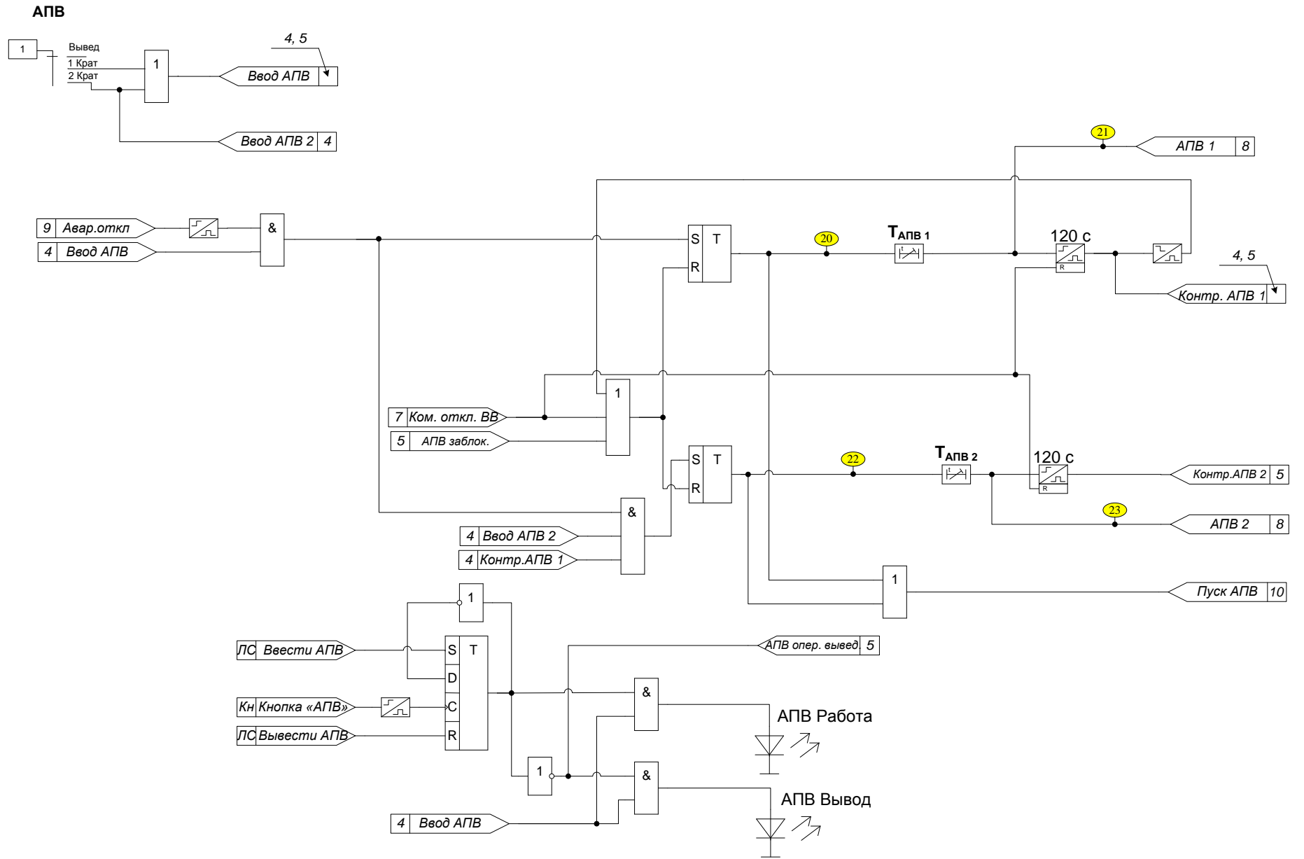
Рисунок Д.4 – Функциональная схема алгоритма АПВ
