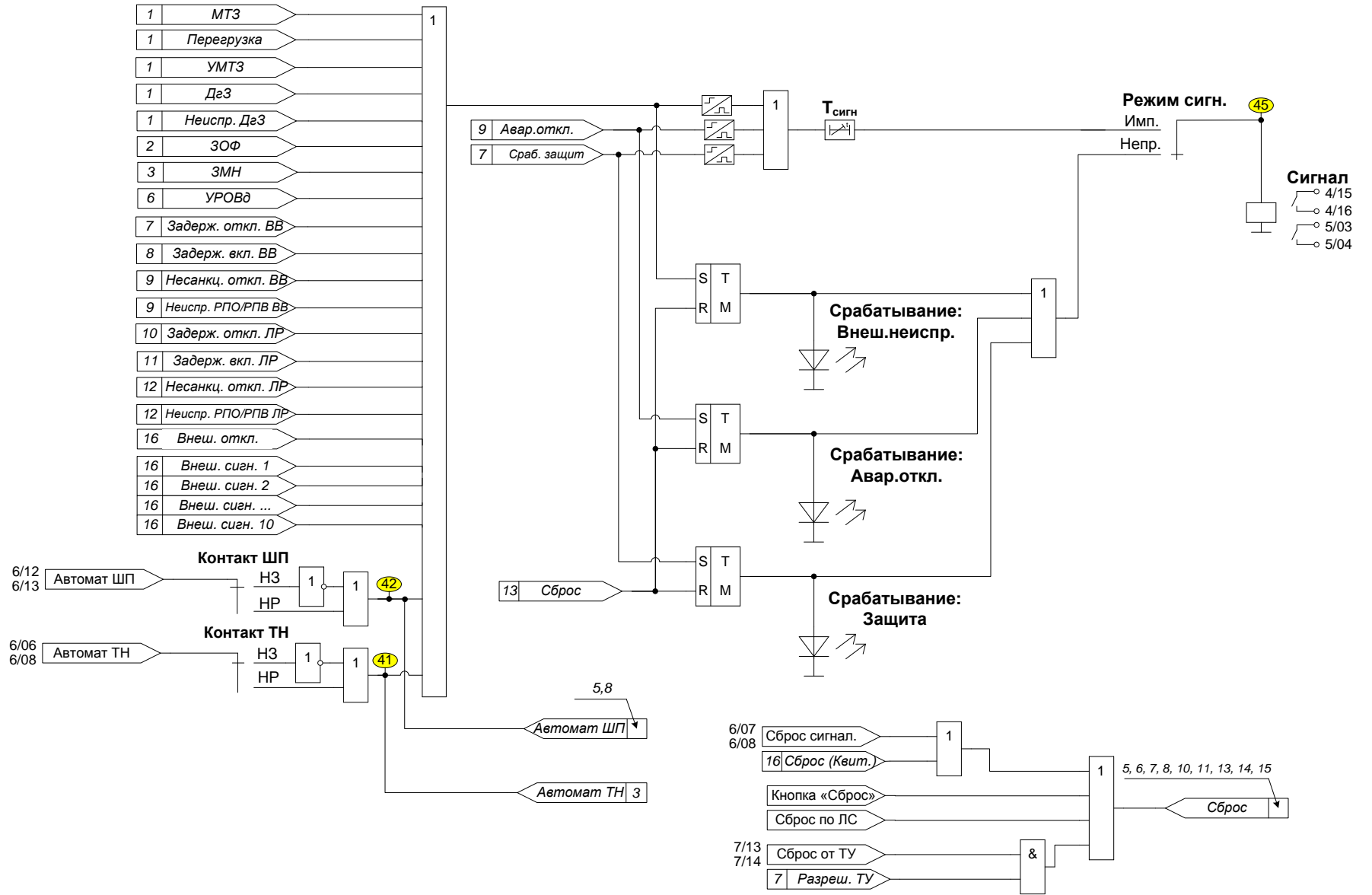
Рисунок Д.13 – Функциональная схема алгоритма сигнализации
