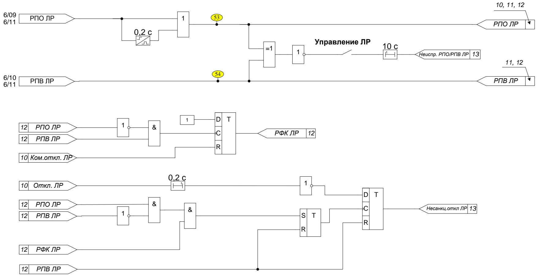
Рисунок Д.12 – Функциональная схема алгоритма диагностики ЛР
