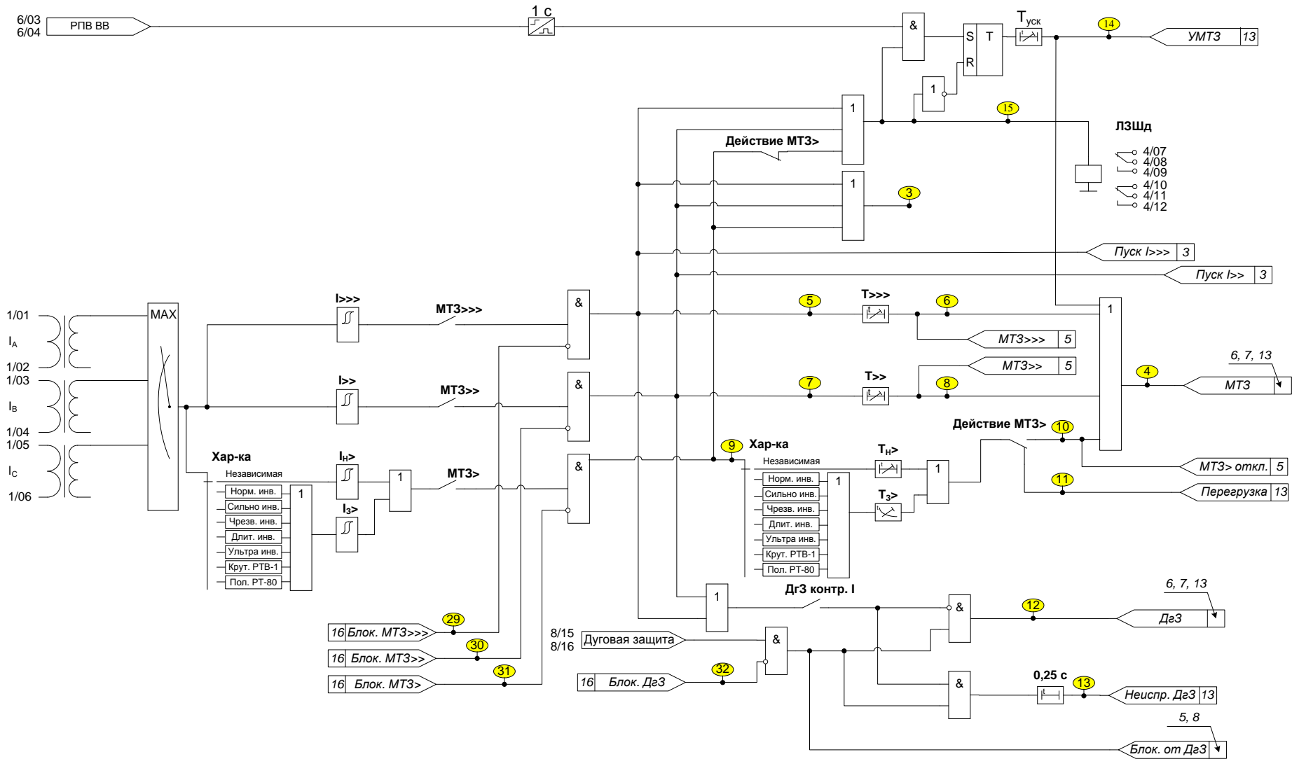
Рисунок Д.1 – Функциональная схема алгоритмов МТЗ, ДгЗ
