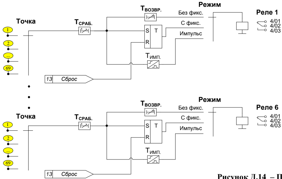
Рисунок Д.14 – Программируемые реле
