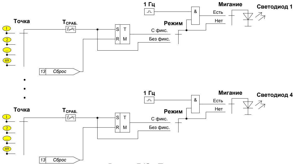
Рисунок Д.15 – Программируемые светодиоды
