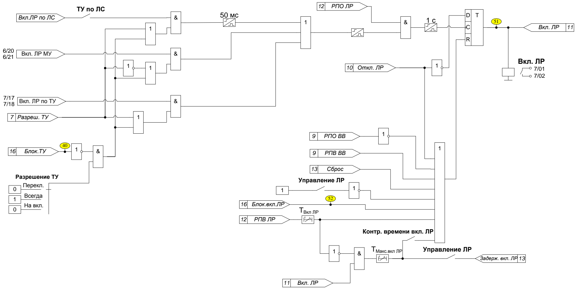
Рисунок Д.11 – Функциональная схема алгоритма включения ЛР
