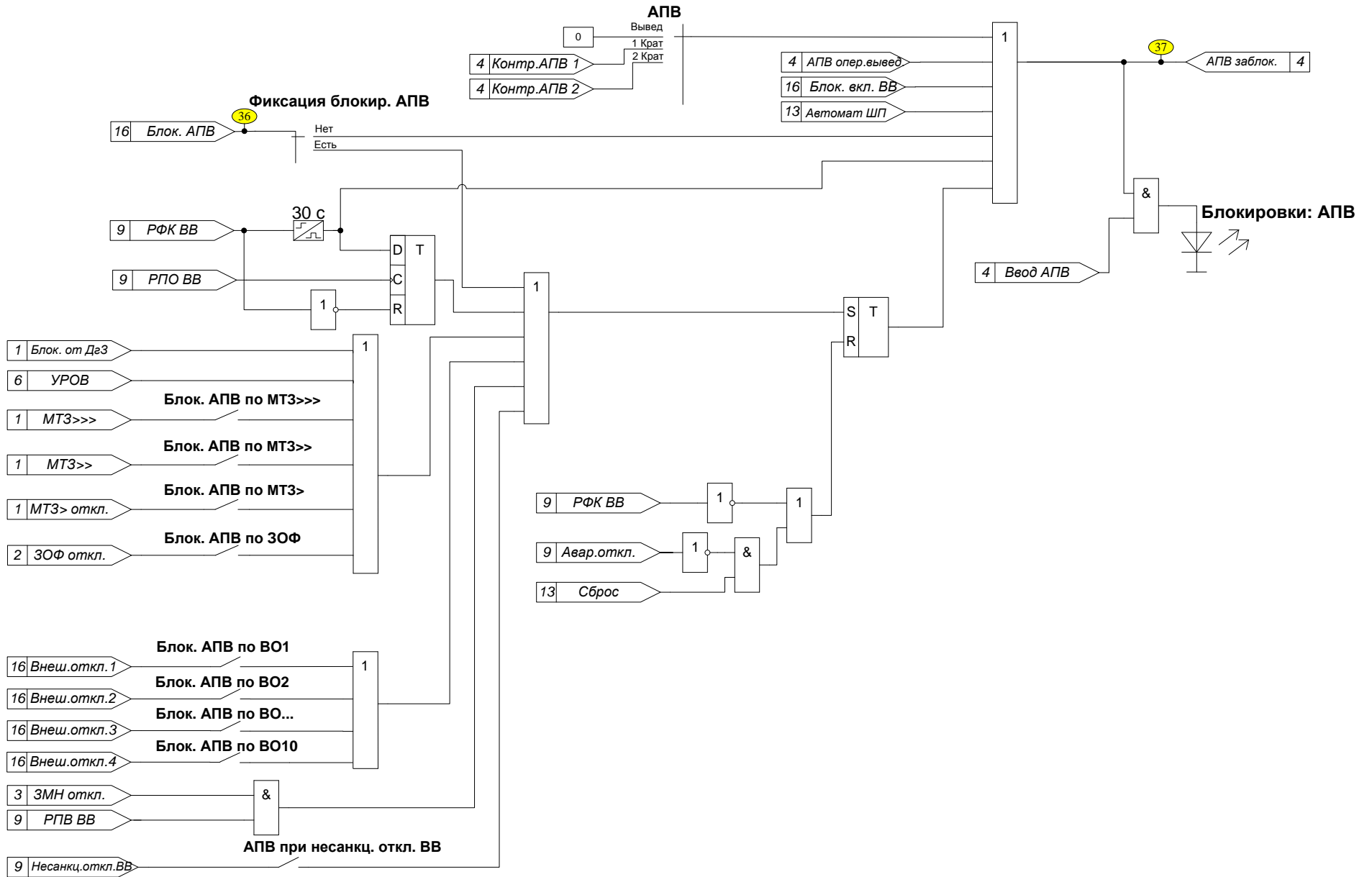
Рисунок Д.5 – Функциональная схема алгоритма блокировки АПВ
