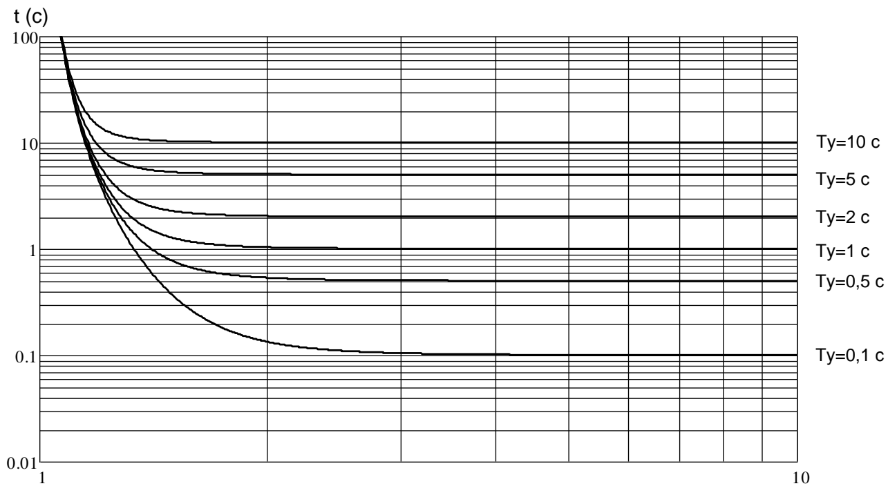
Рисунок Е.7 – Крутая характеристика (аналог РТВ-1)
