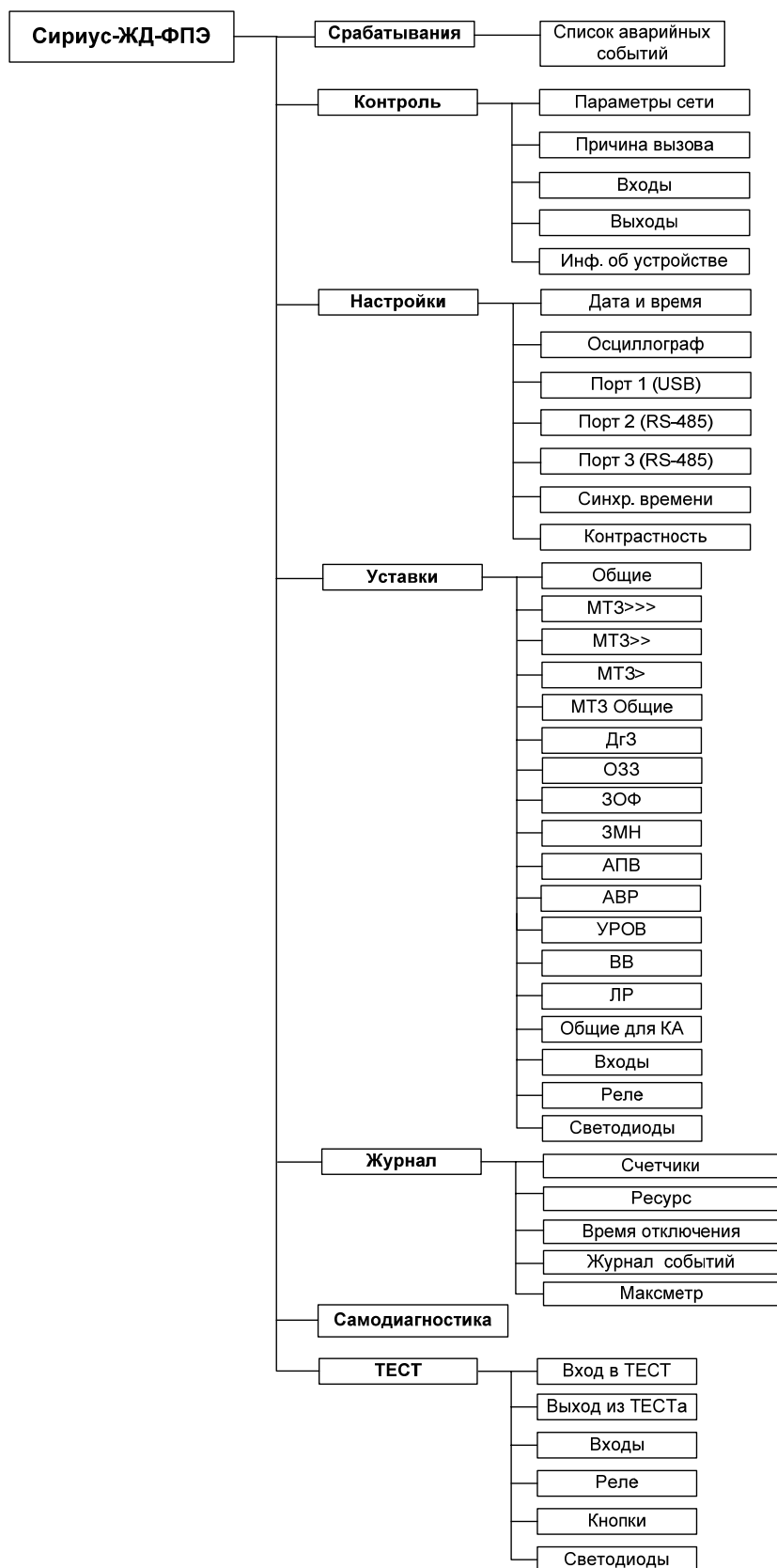
Рисунок Г.1 – Общая структура меню (пример)
