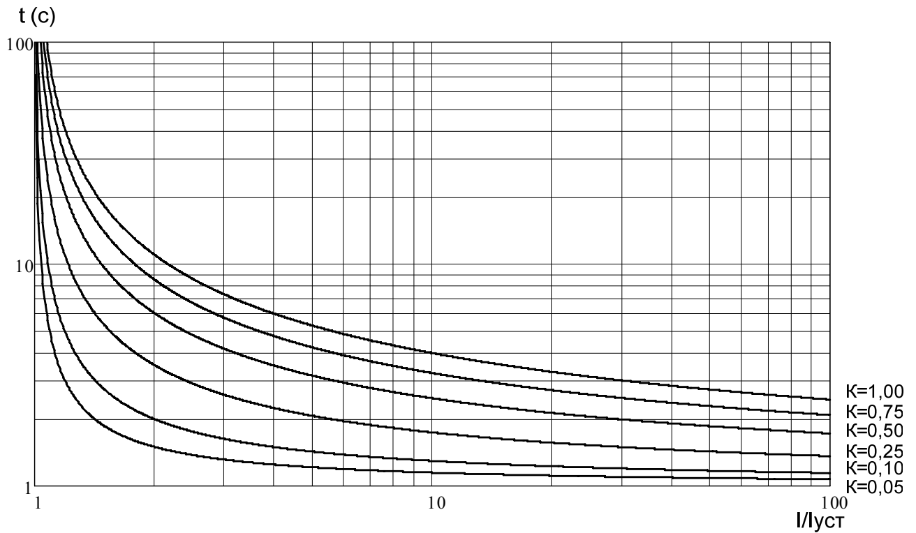
Рисунок Е.1 – Нормально инверсная характеристика по МЭК 255-4
