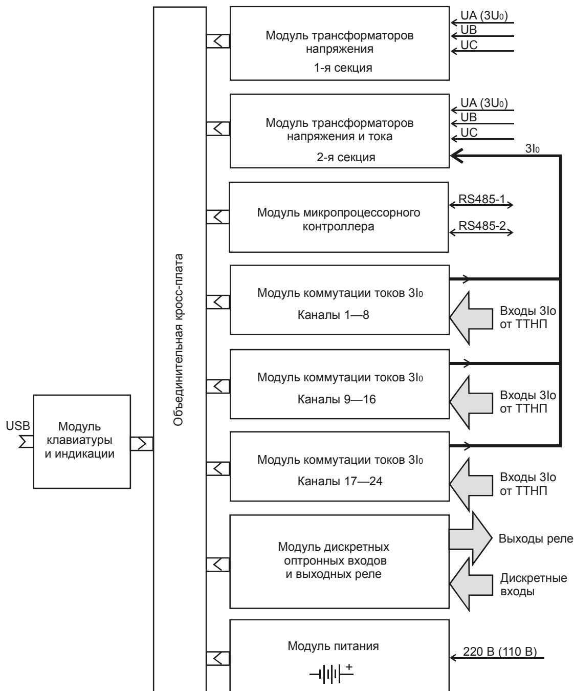
Рисунок 2 – Структурная схема устройства «Сирius-033»
