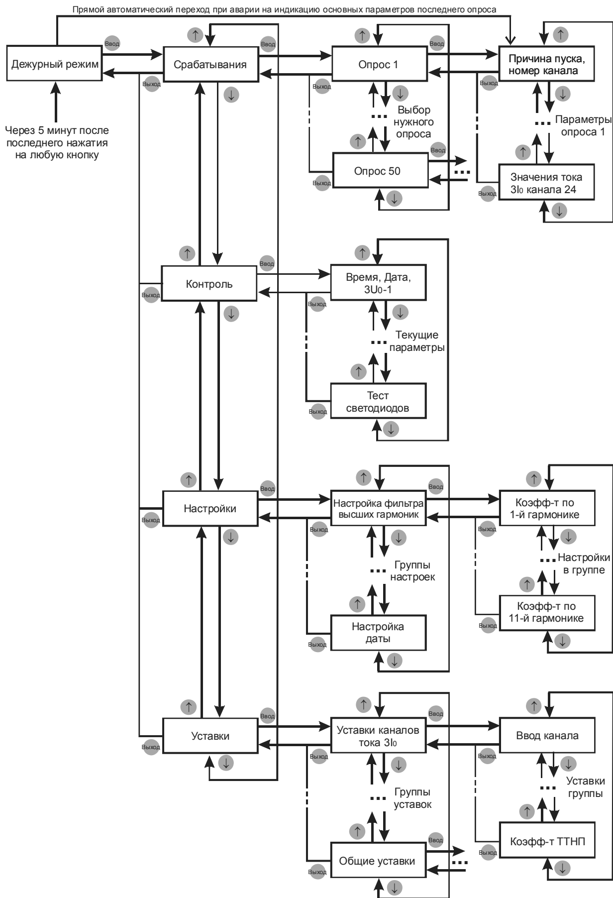
Рисунок 3 – Общая структура диалога с устройством «Сириус-033»
