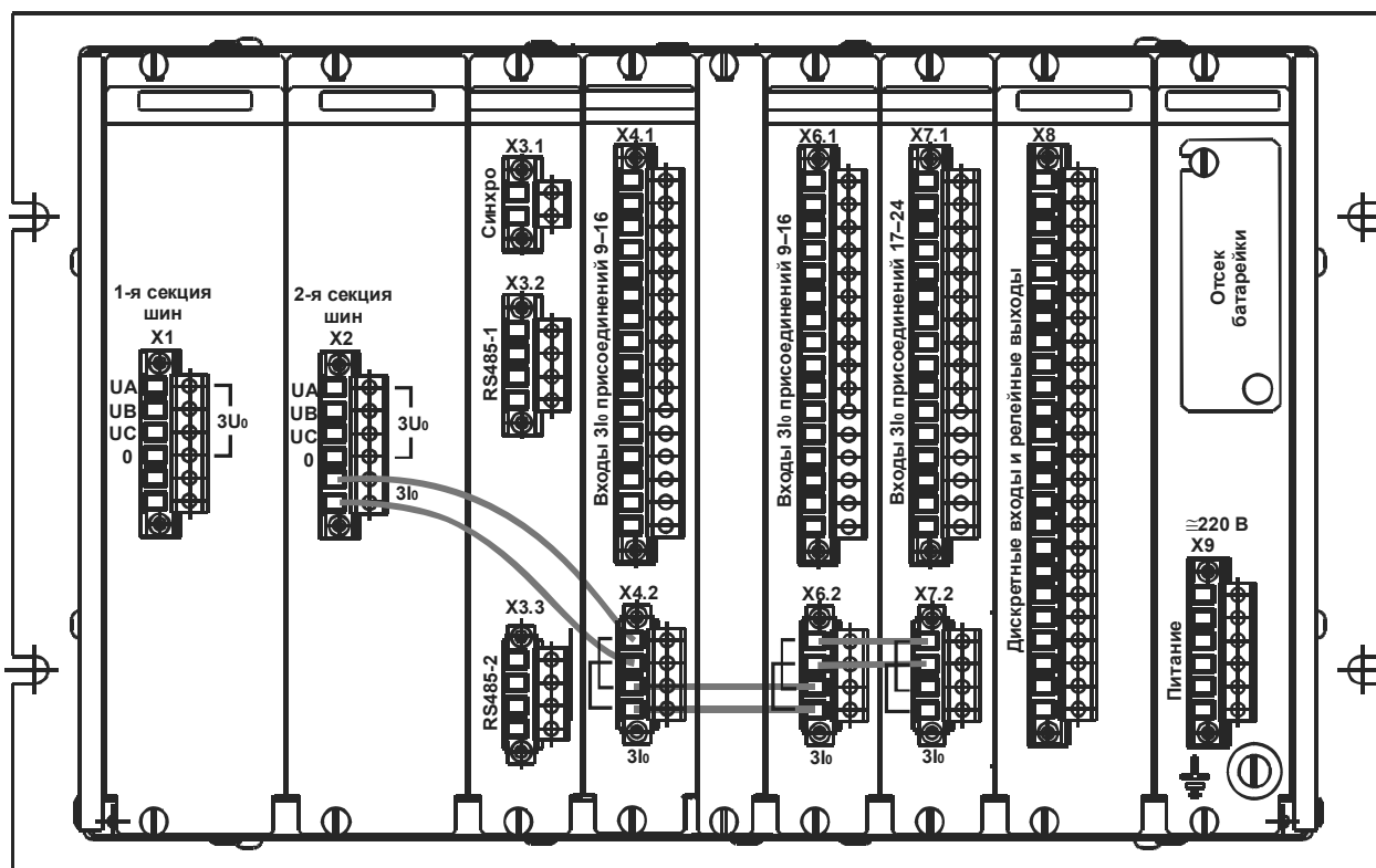
Рисунок Б.2 – Вид сзади
