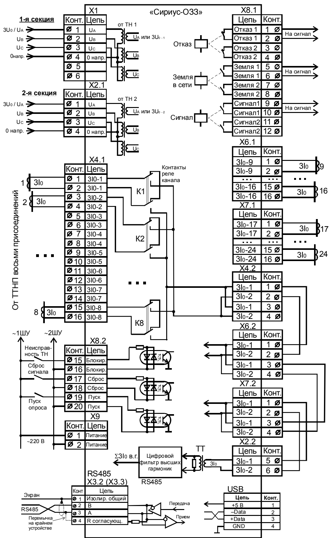
Рисунок В.1 – Схема подключения устройства «Сириус-ОЗЗ» к внешним цепям
