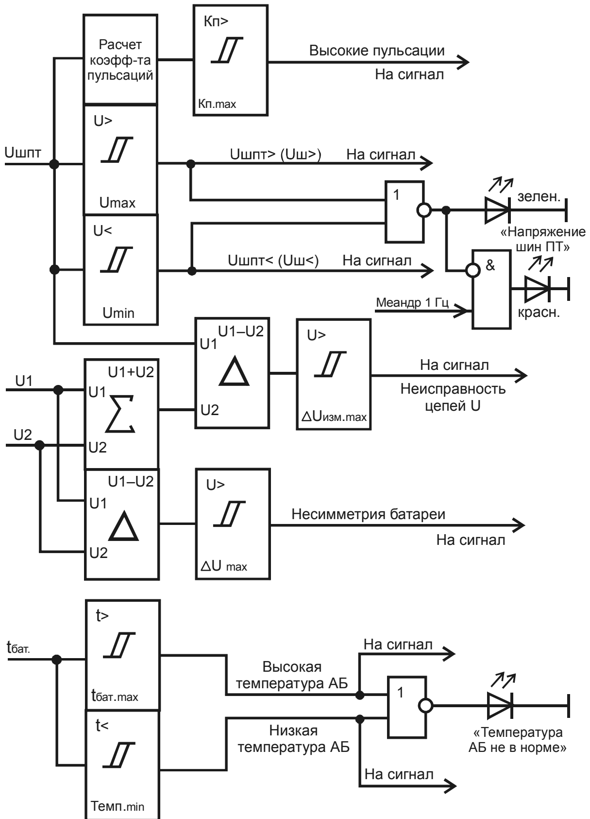
Рисунок Ж.5 – Фрагмент функциональной логической схемы обработки сигналов напряжения и температуры
