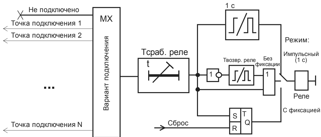
Рисунок Ж.2 – Программируемые реле
