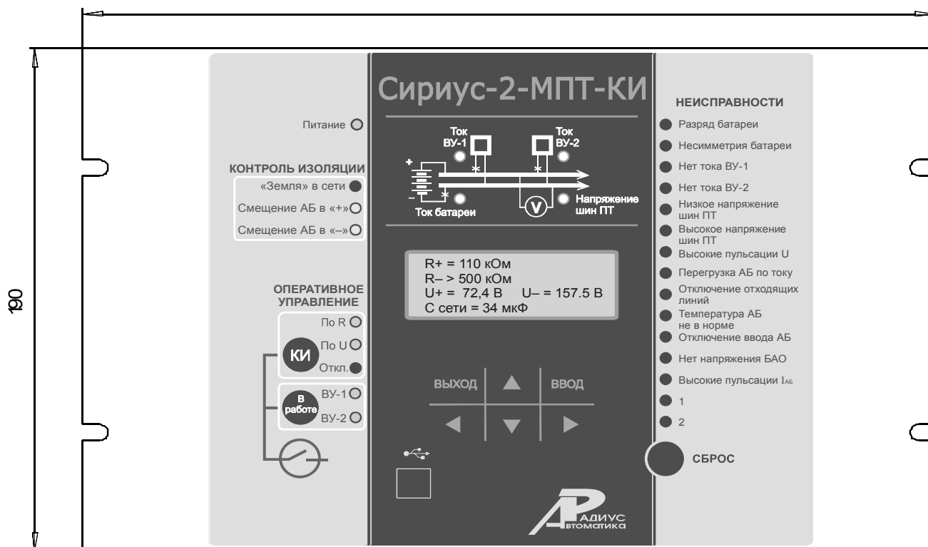
Рисунок Г.1 – Вид спереди
