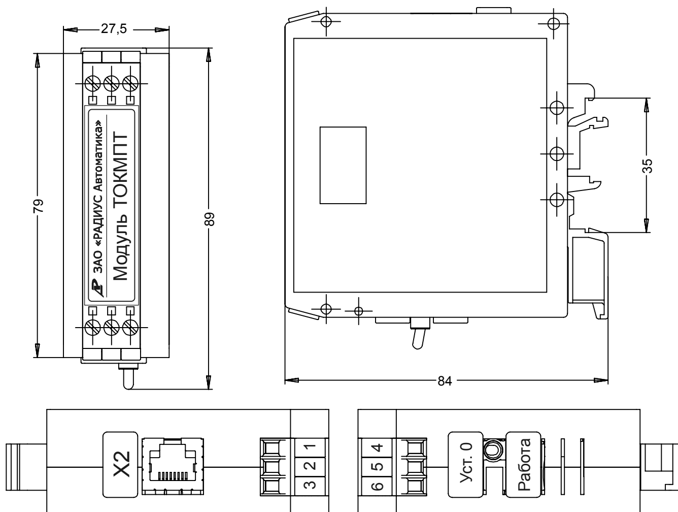
Рисунок Г.6 – Модуль тока ТОКМПТ
