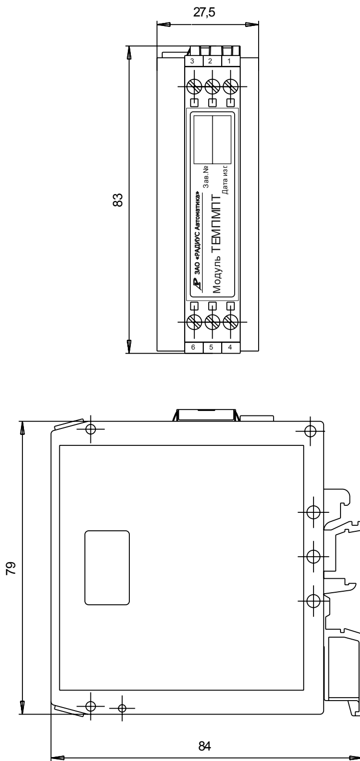
Рисунок Г.7 – Модуль датчика температуры ТЕМПМПТ
