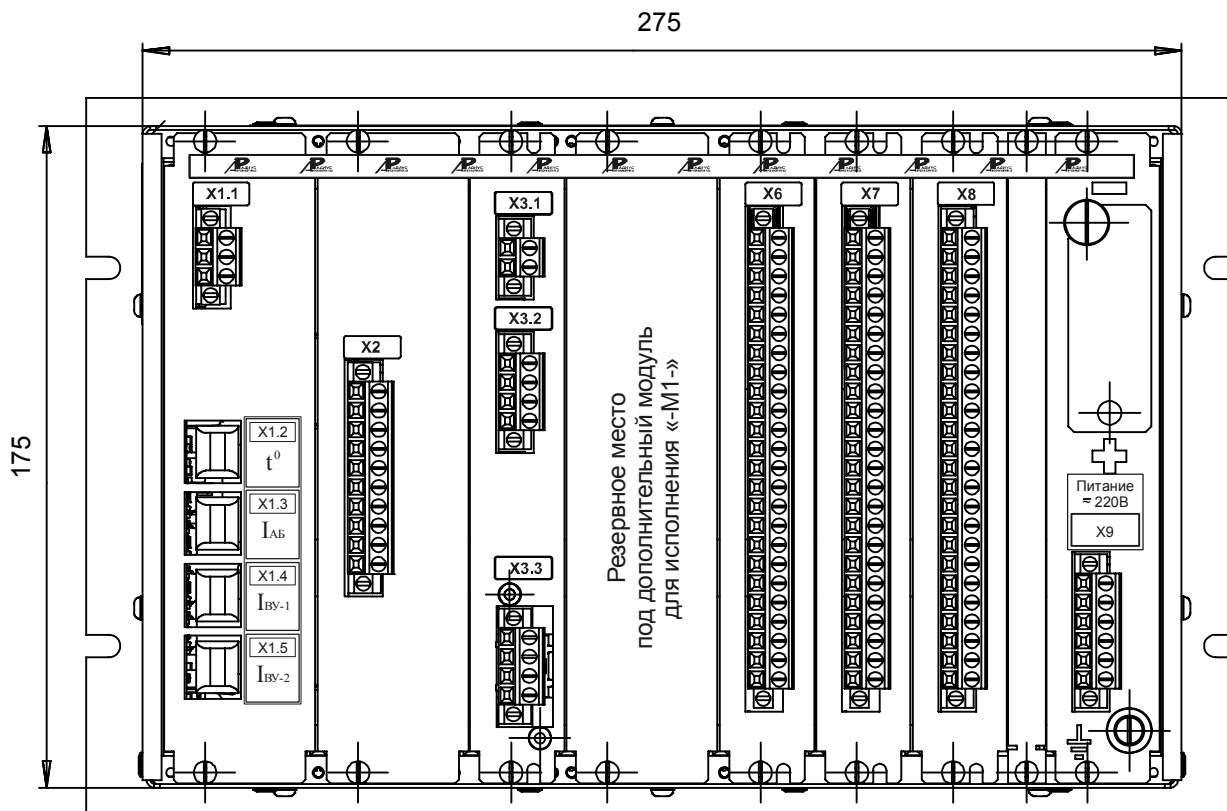
Рисунок Г.4 – Расположение элементов на задней панели устройства «Сириус-2-МПТ-КИ» (показано исполнение «-М0-И1»)
