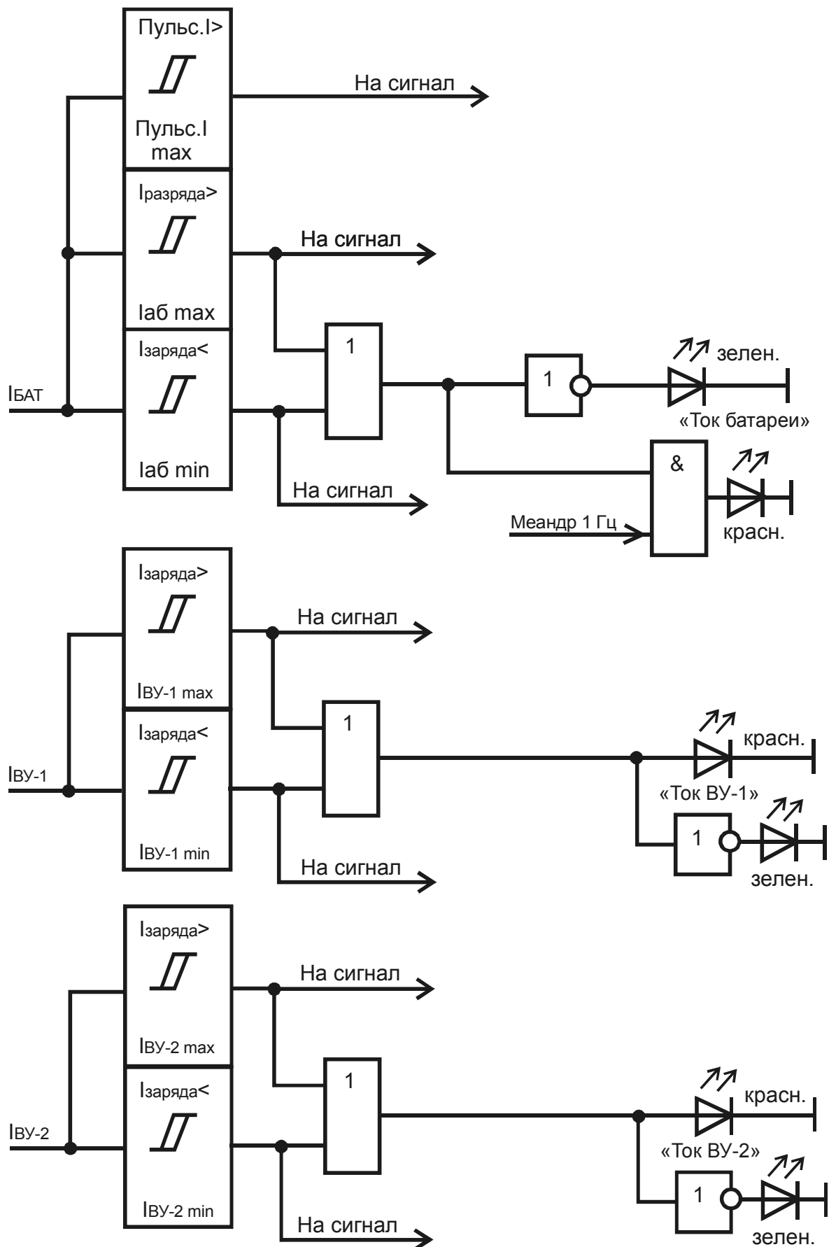
Рисунок Ж.6 – Фрагмент функциональной логической схемы обработки сигналов тока
