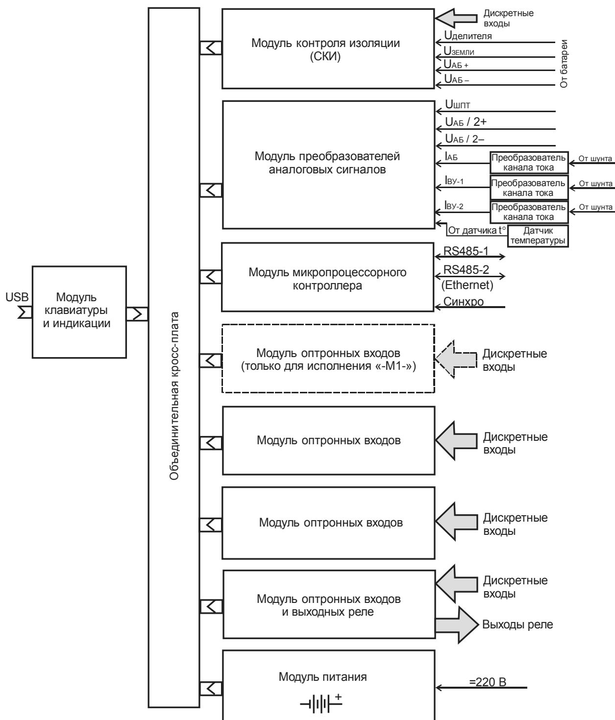
Рисунок 1.1 – Структурная схема устройства
