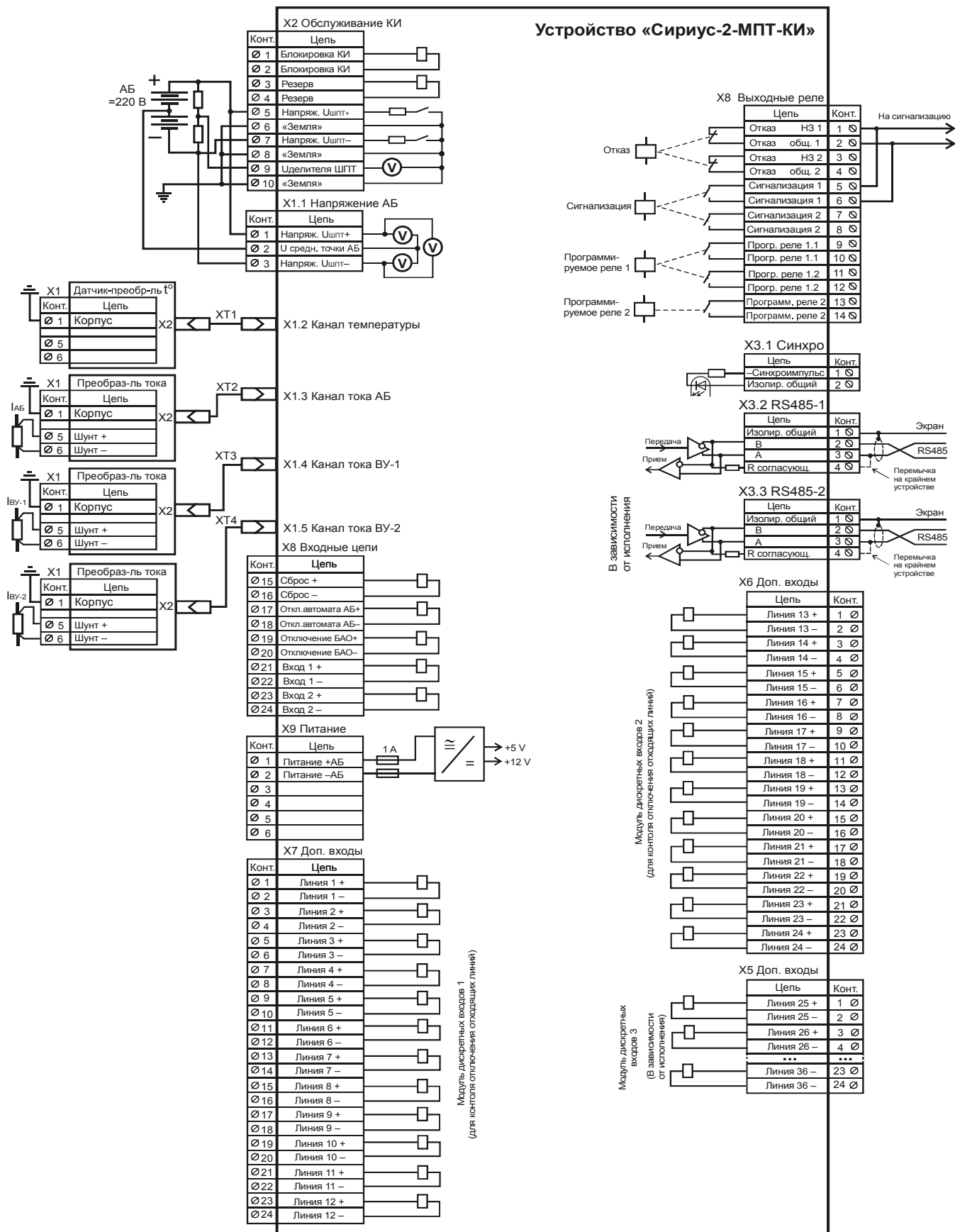
Рисунок Д.1 – Схема подключения внешних цепей к устройству «Сириус-2-МПП-КИ»
