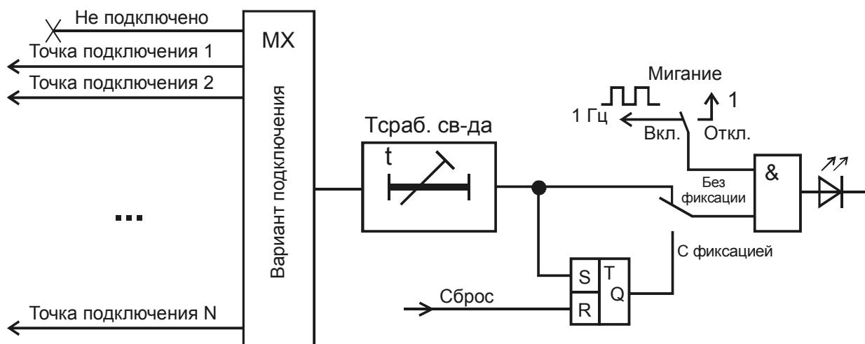
Рисунок Ж.3 – Программируемые светодиоды
