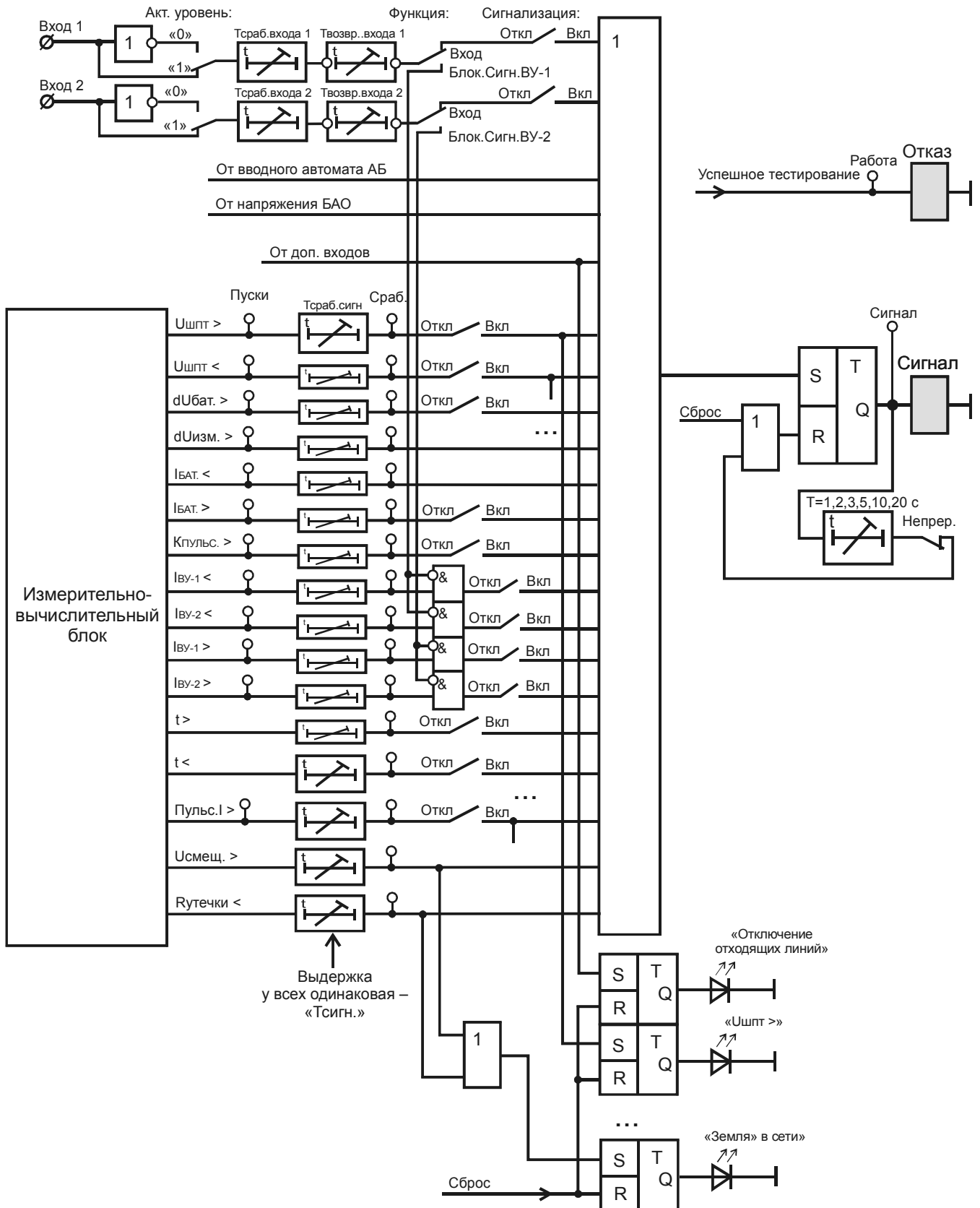
Рисунок Ж.4 – Фрагмент функциональной логической схемы выходного реле «Сигнал»
