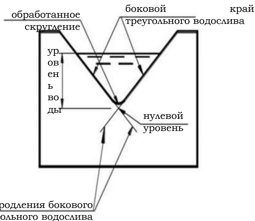
Рисунок 7.1.2 Установка треугольного водослива в канале и нулевой уровень треугольного водослива
