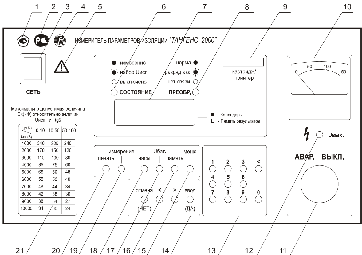
Рисунок 3. Внешний вид лицевой панели блока управления
