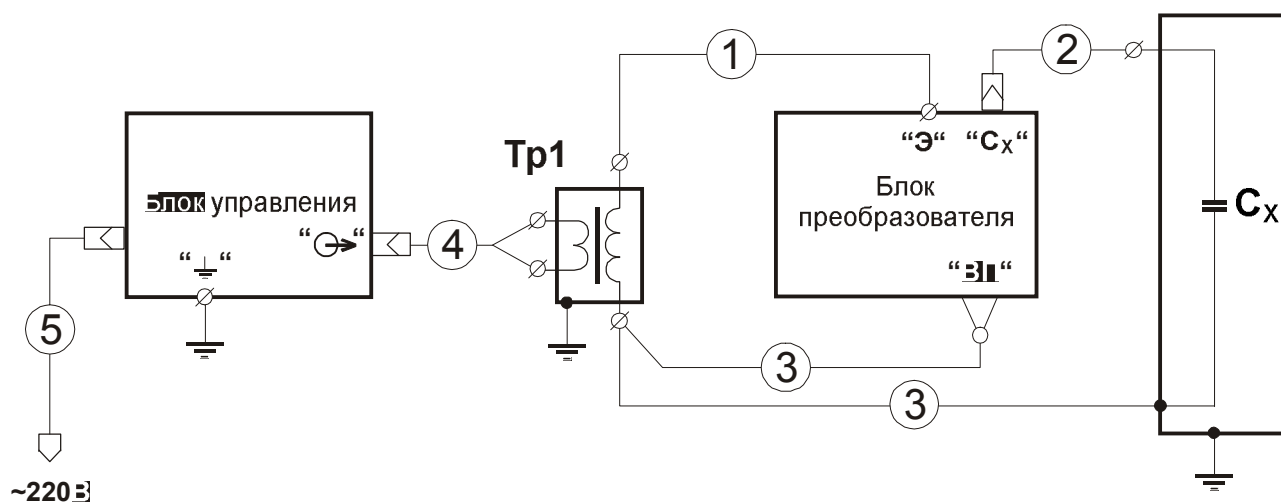
Рисунок 2. «Перевернутая» схема измерений.
