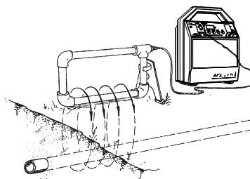
Индуктивное подключение
