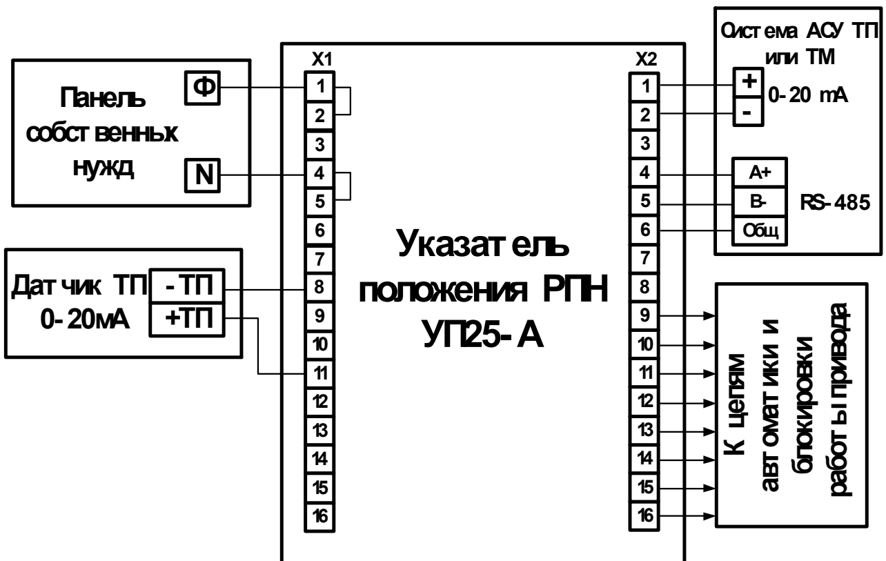
Рис. 3.3 Схема привязки УП 25-А к датчику «Токовая петля» 0-20 мА.
