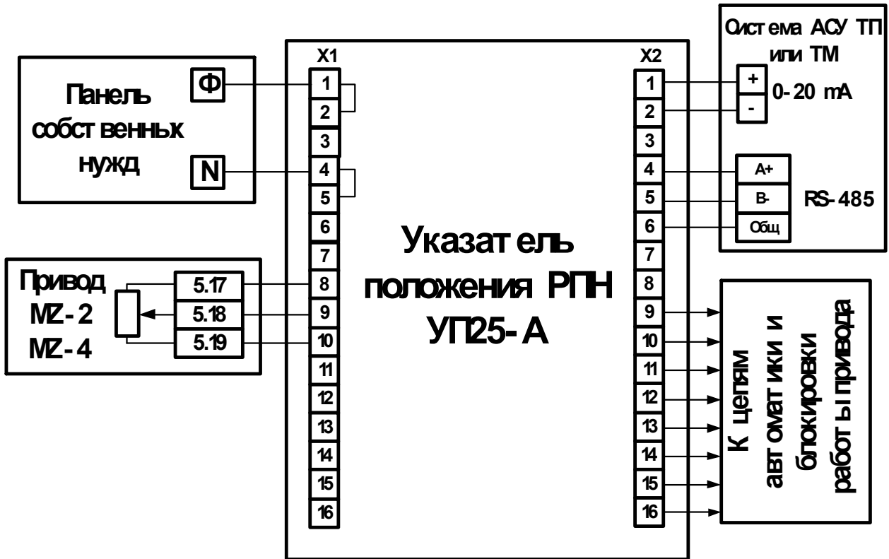
Рис. 3.2 Схема привязки УП 25-А к приводу типа MZ-2, MZ-4.
