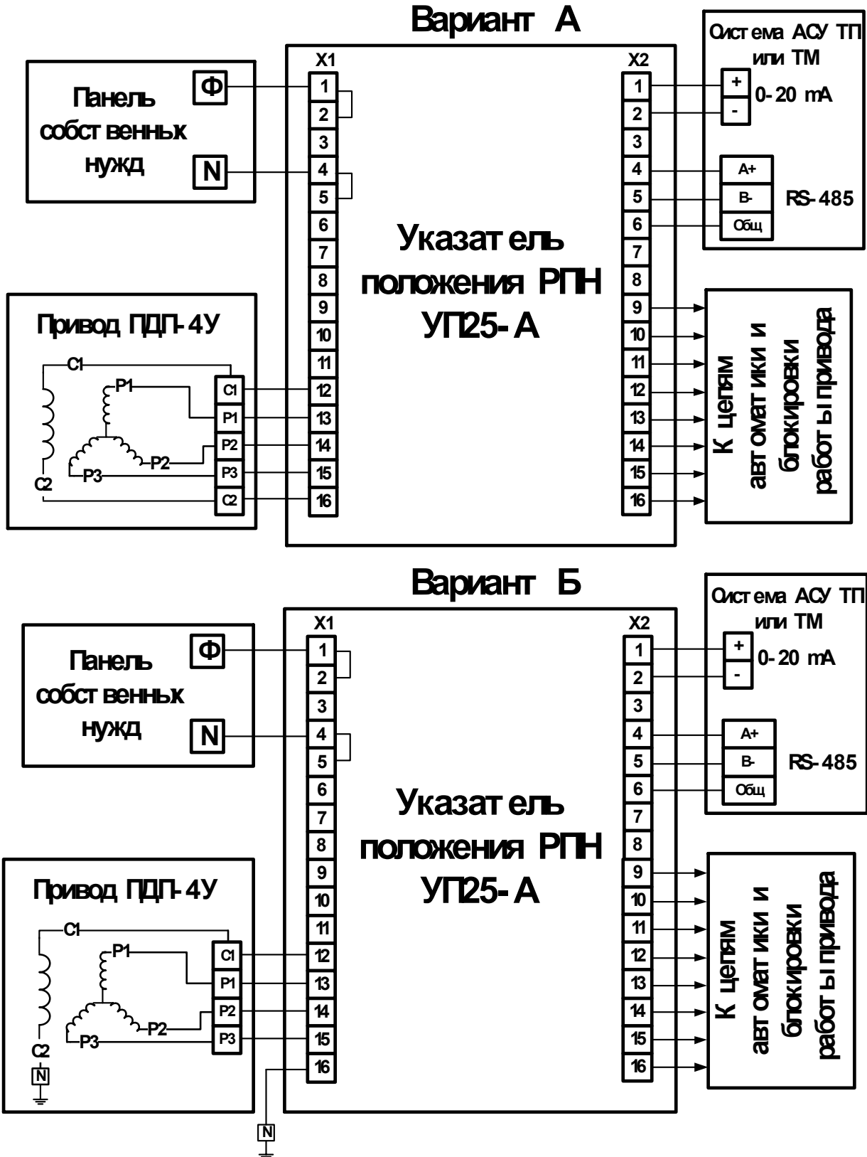
Рис. 3.1 Схемы привязки УП 25-А к приводу типа ПДП-4У.
