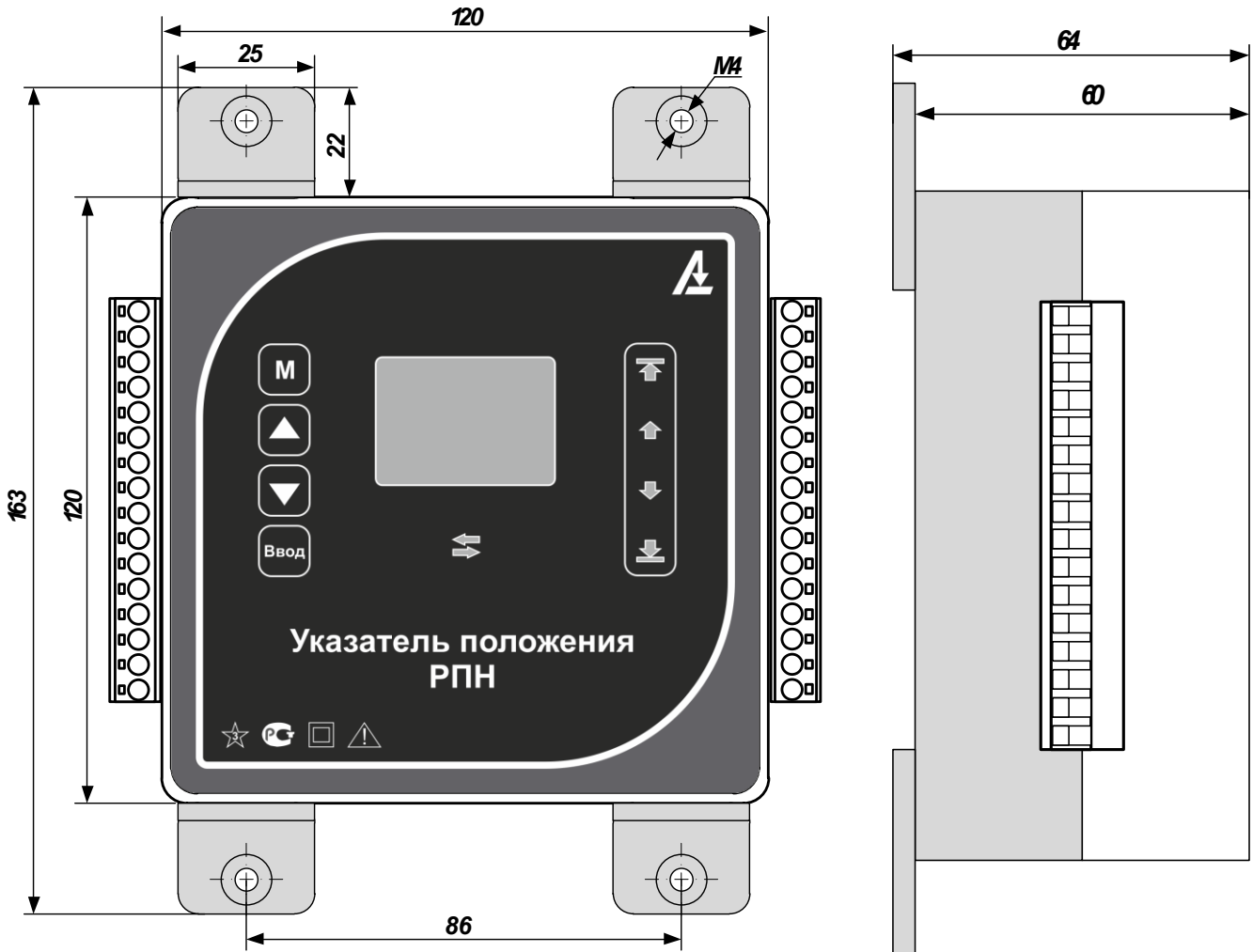
Рис. 1.1 Габаритные размеры указателя положения РПН УП 25-А (настенный вариант).
