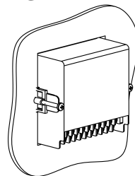
Рисунок 4.9 – Монтаж прибора в корпусе Щ11
