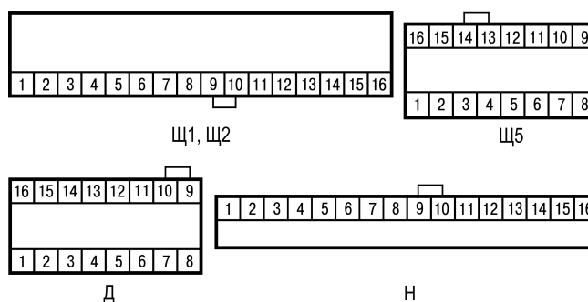
Рисунок 7.8 – Установка переключки
