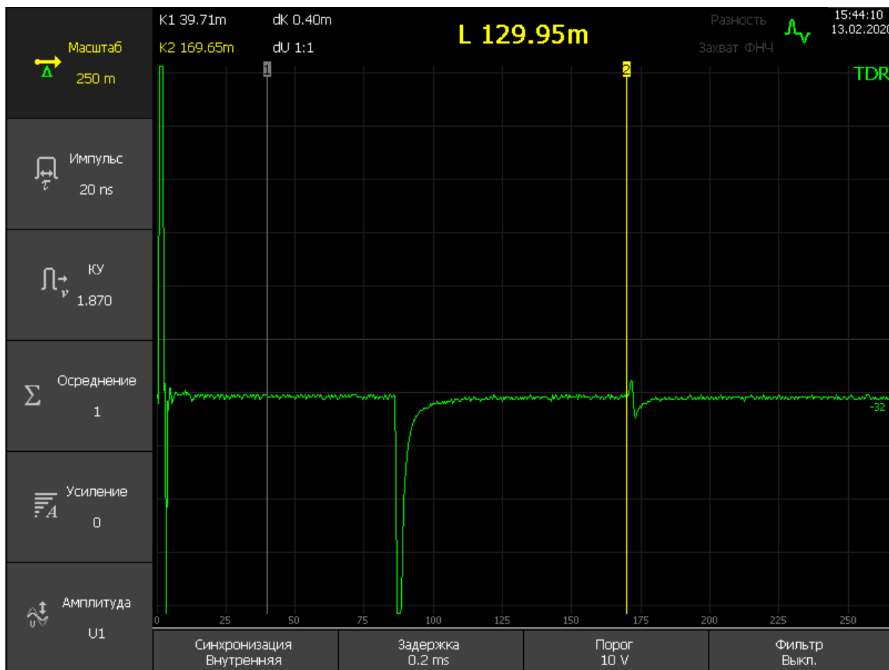
Рисунок 4.8. Окно «ПАРАМЕТРЫ»
